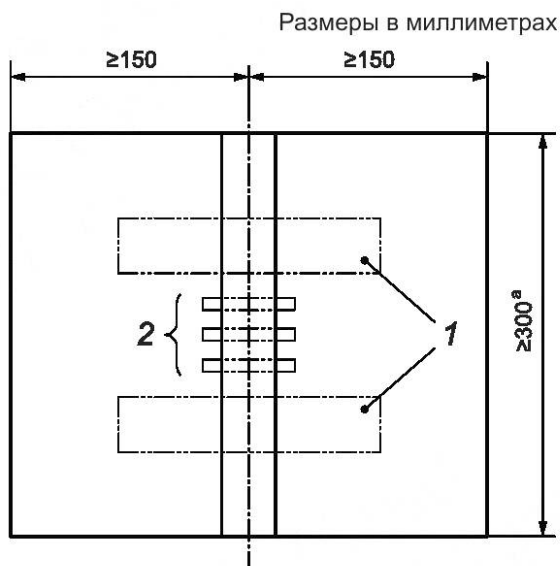
а) Расположение образцов для испытаний на поперечное растяжение и ударный изгиб (при односторонней сварке)
