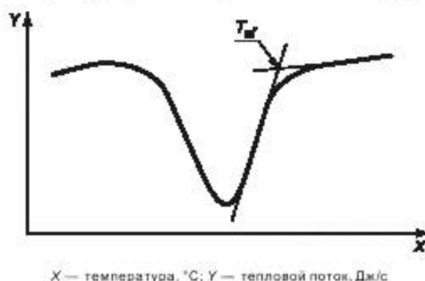
Рисунок 2 — Кривая дифференцирующей сканирующей калориметрии
