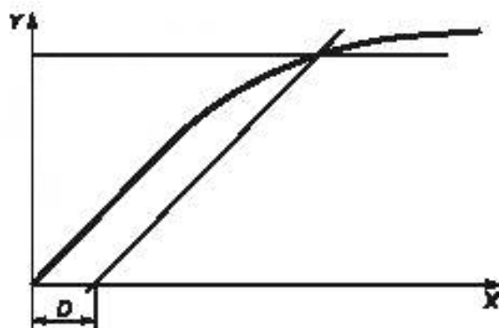
Рисунок 4 — График жесткости при изгибе
