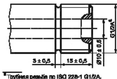
Рисунок 1 — Входной порт для клемм датчика температуры
