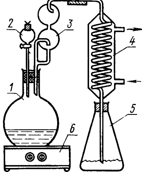
1—дистилляционная колба; 2—капельная воронка; 3—дефлегматор; 4—холодильник; 5—приемная колба; 6—электроплитка.
