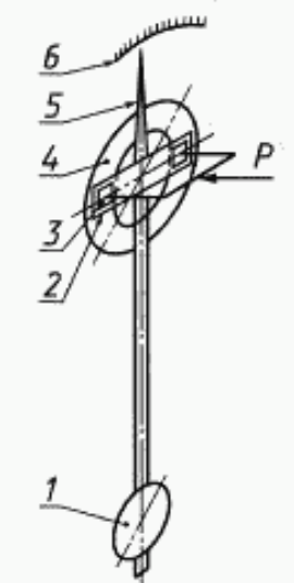
1 — маятник; 2 — держатель образцов; 3 — образцы; 4 — металлическое контртелo; 5 — стрелка; 6 — шкала момента трения
