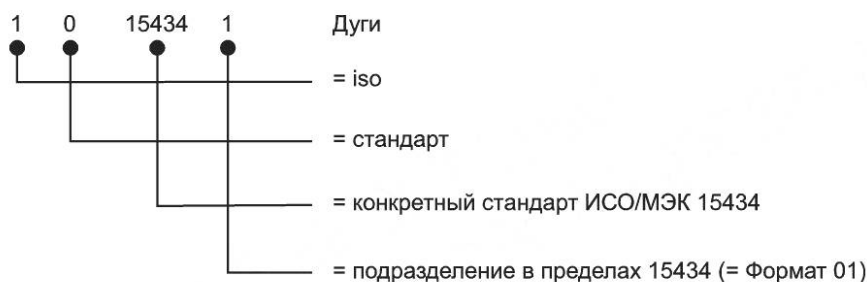
Рисунок 2 — Пример дуг идентификатора объекта
