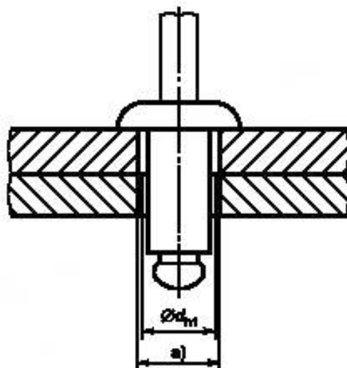
а) Увеличенное отверстие с зазором.
