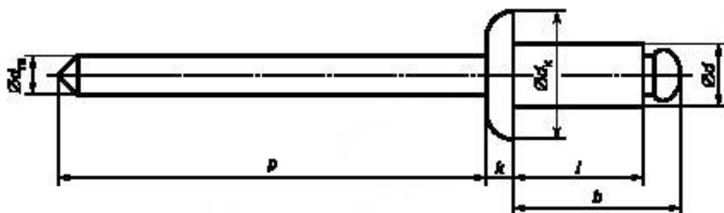
Рисунок 1 — Размеры заклепок
