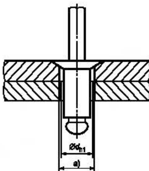
а) Увеличенное отверстие с зазором.
