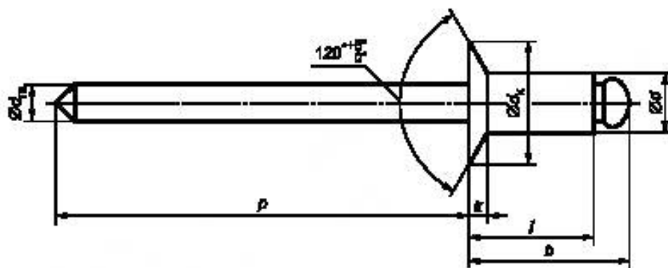
Рисунок 1 — Размеры заклепок
