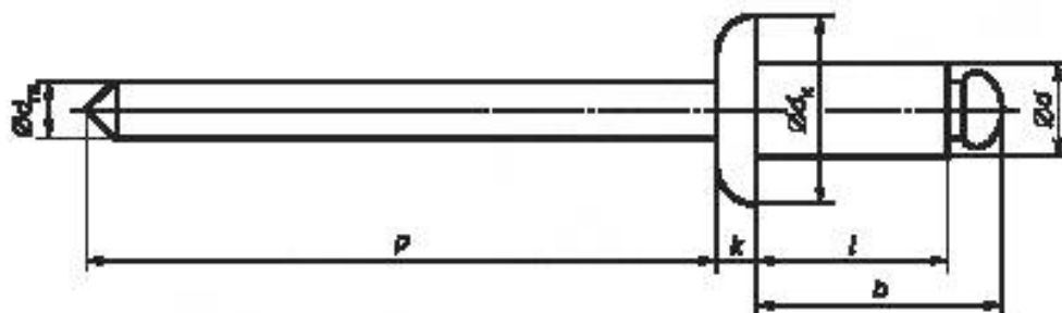
Рисунок 1 — Размеры заклепок
