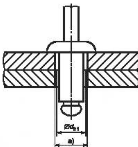
Рисунок 2 — Увеличенное отверстие с зазором для облегчения совмещения
