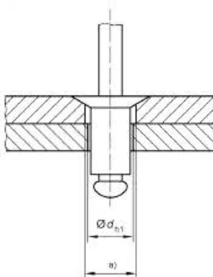
Рисунок 2 — Увеличенное отверстие с зазором для облегчения совмещения
