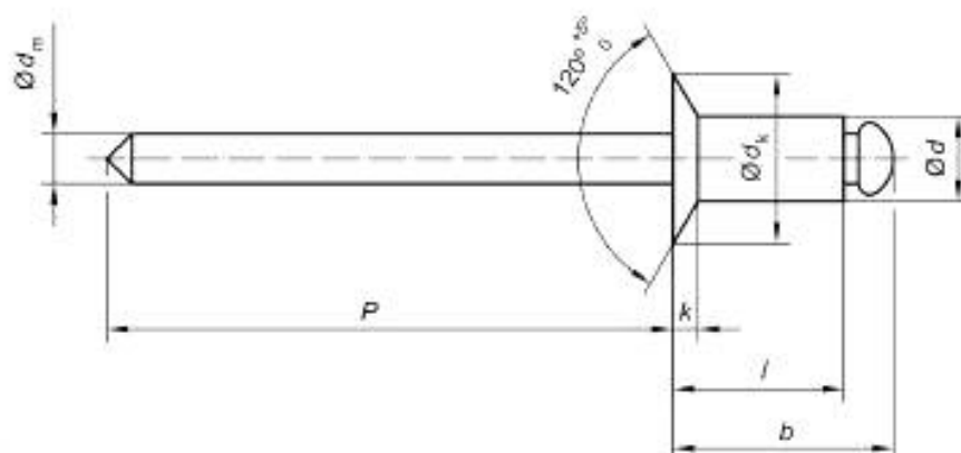
Рисунок 1 — Размеры заклепок
