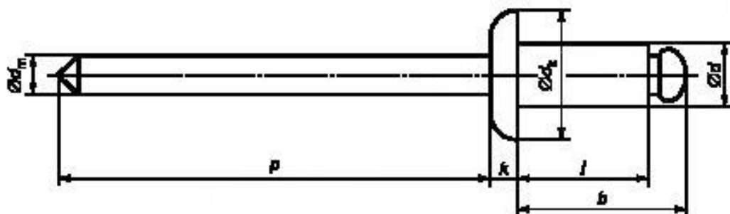
Рисунок 1 — Размеры заклепок
