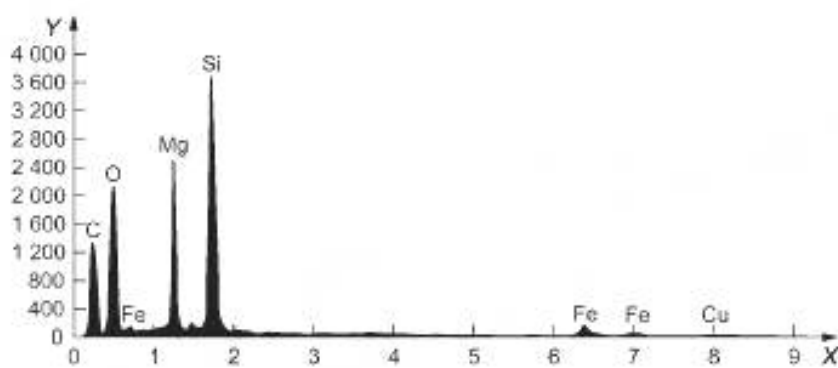
f) Антофиллит (без покрытия золотом)
