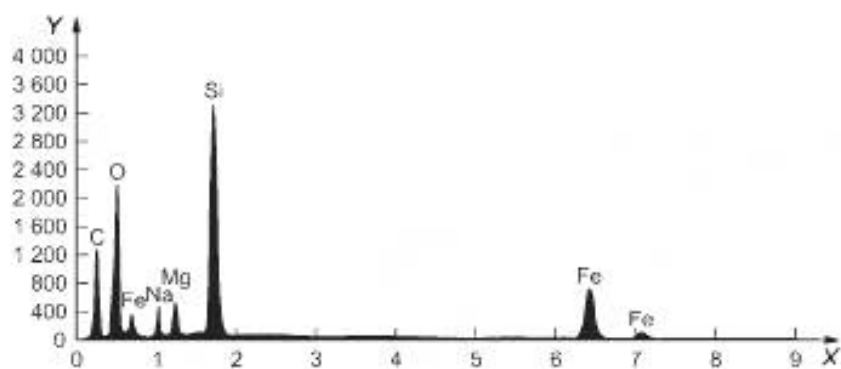
с) Крокидолит (без покрытия золотом)
