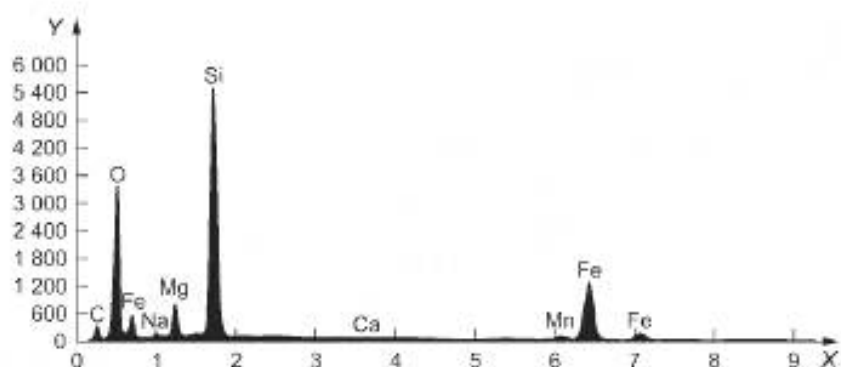
б) Амозит (без покрытия золотом)
