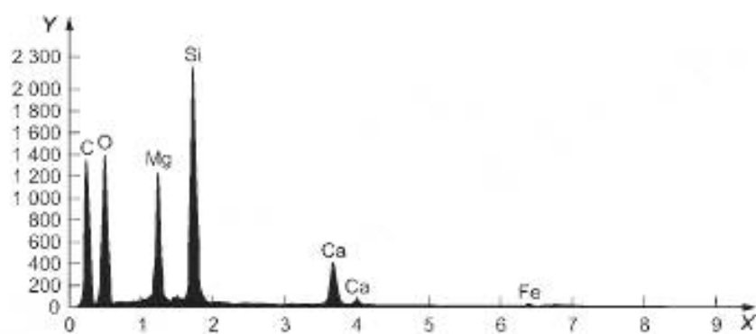
d) Тремолит (без покрытия золотом)
