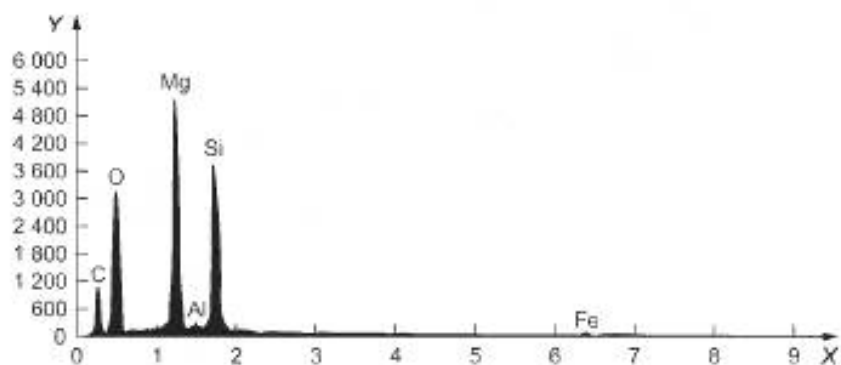
а) Хризотил (без покрытия золотом)
