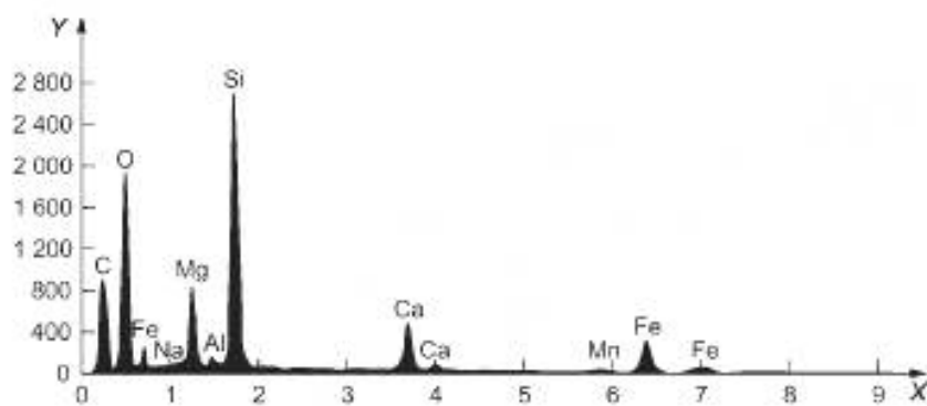
e) Актинолит (без покрытия золотом)
