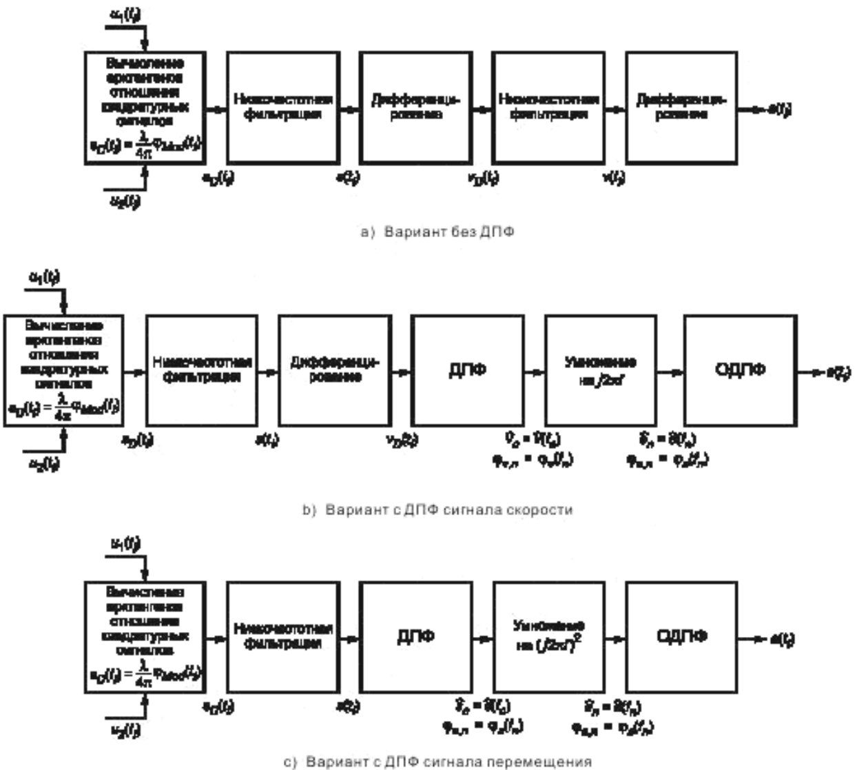
Рисунок 4 — Блок-схема обработки сигнала для получения коэффициента преобразования по удару
