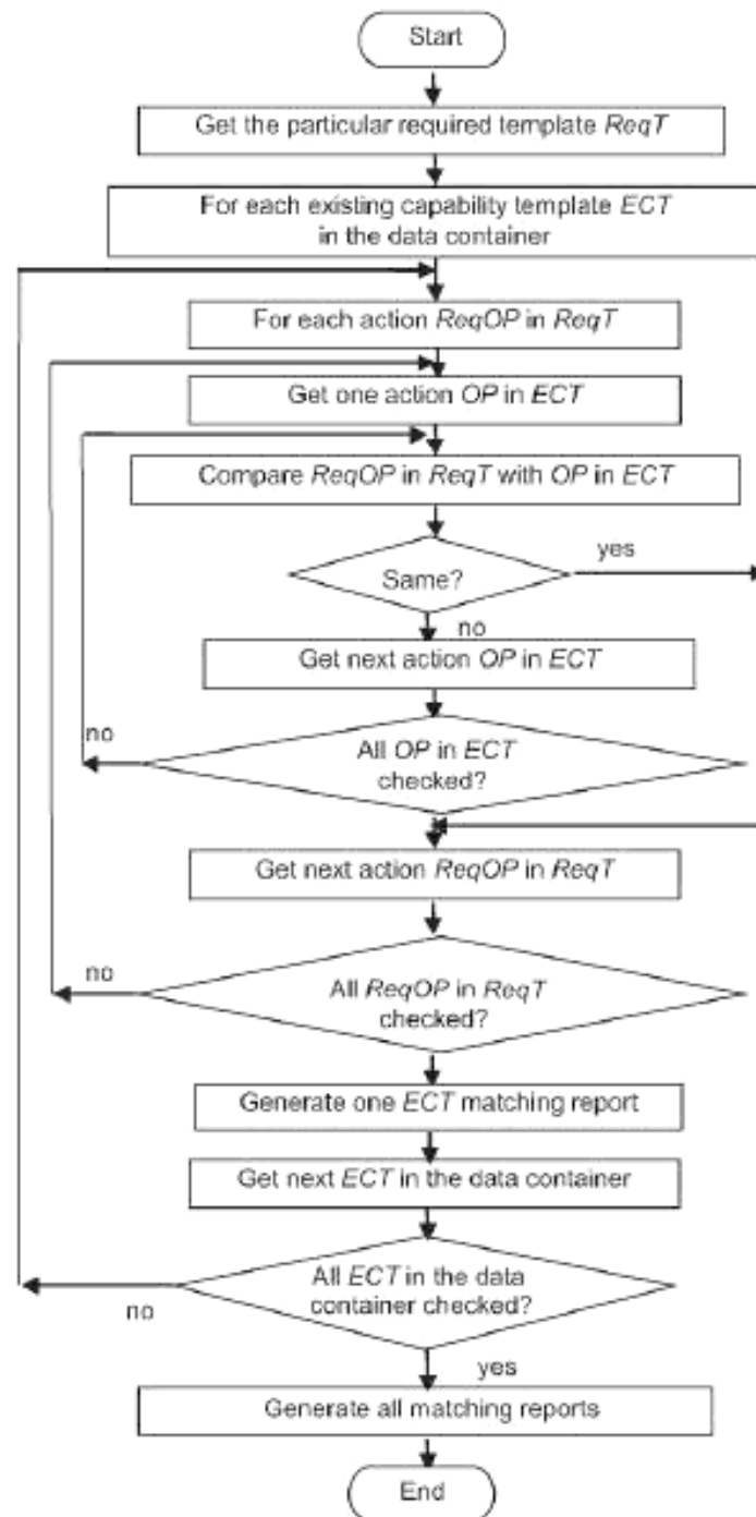
Рисунок В.2 — Процедура выбора шаблона профиля возможностей из Архива
