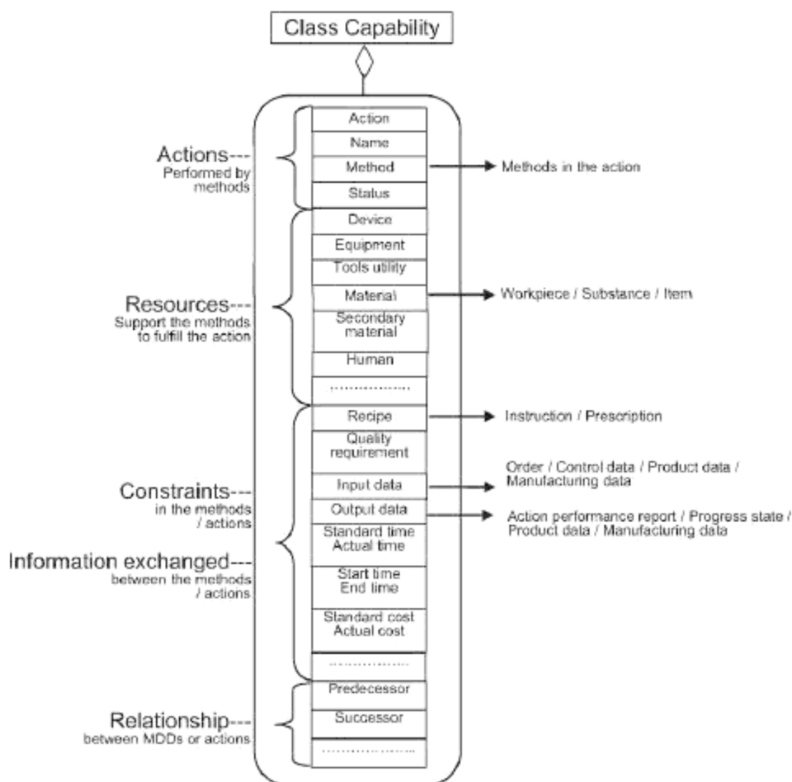
Рисунок А.1 — Отображение модели возможностей на модель производственной деятельности с помощью объектов данных MDD
