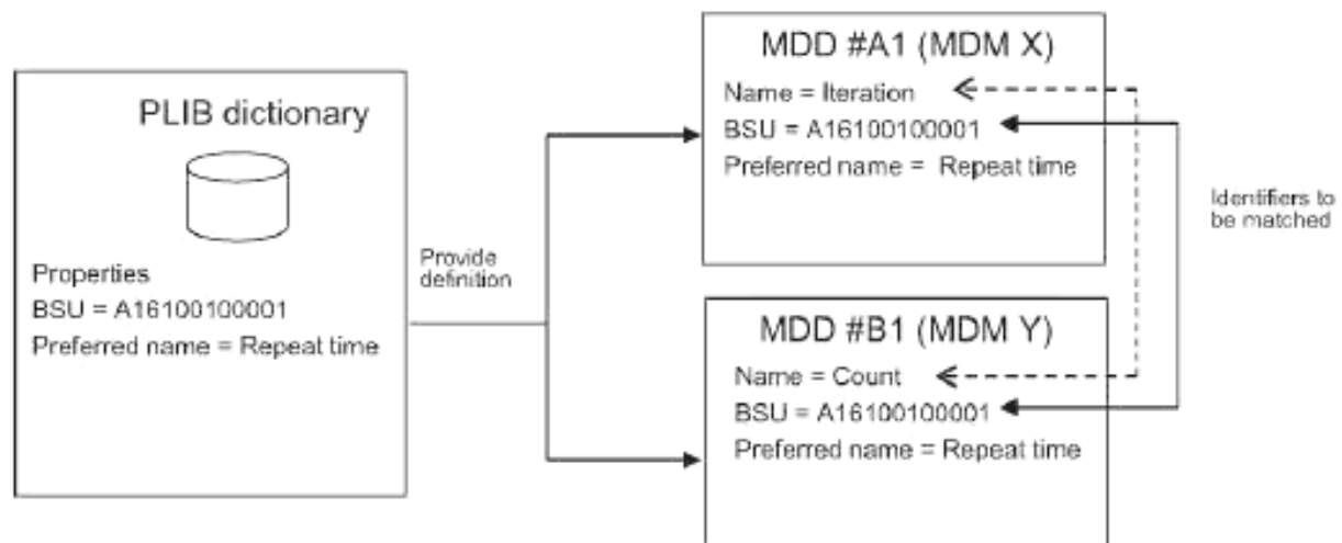
Рисунок E.2 — Сравнение объектов MDD, используя идентификаторы понятий PLIB
