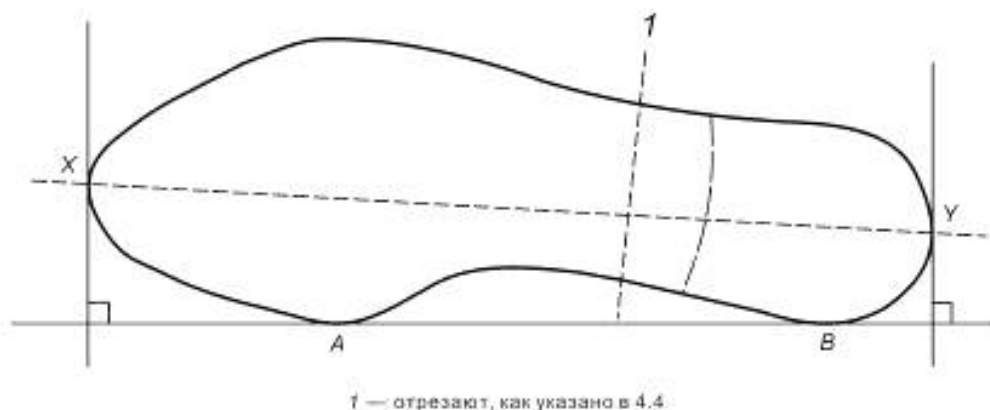
Рисунок 1 — Маркировка и разрез испытуемого образца (см. также рисунок 42 [2])
