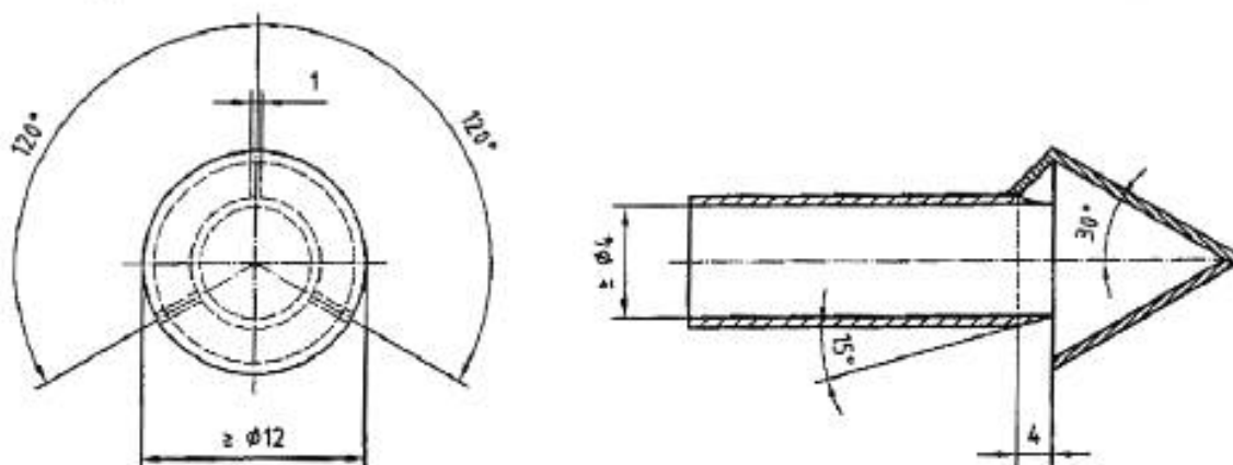
Рисунок 12 – Пробоотборник с коническим наконечником
