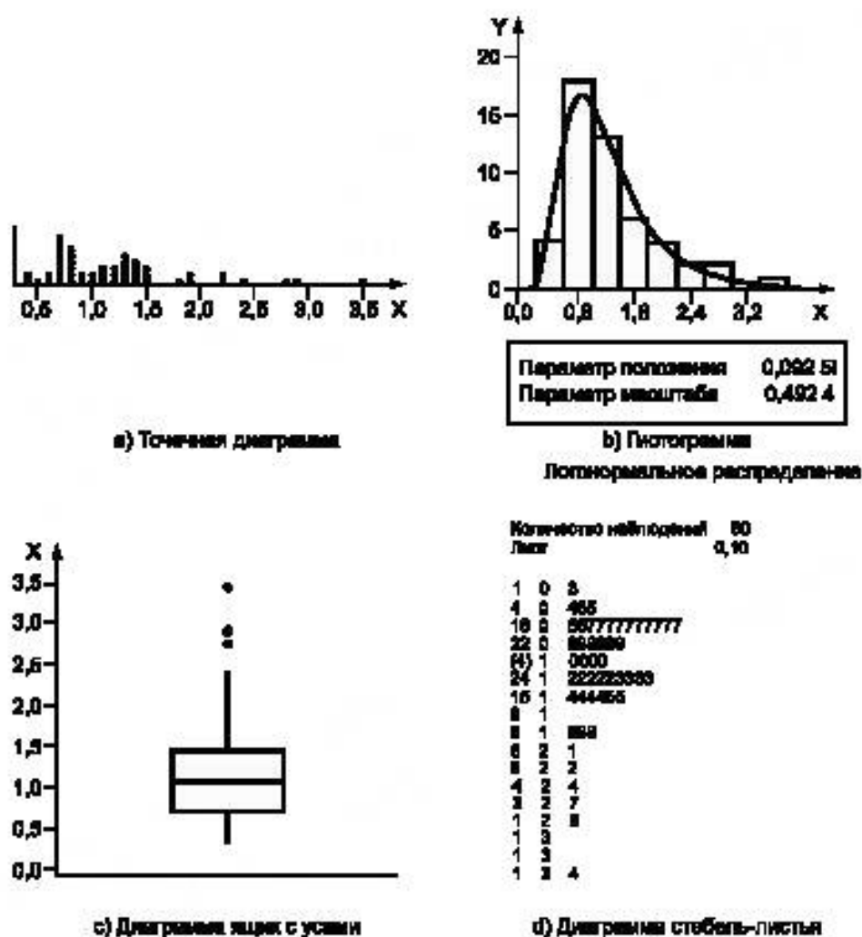
Рисунок 3 — Диаграммы, построенные по набору данных
