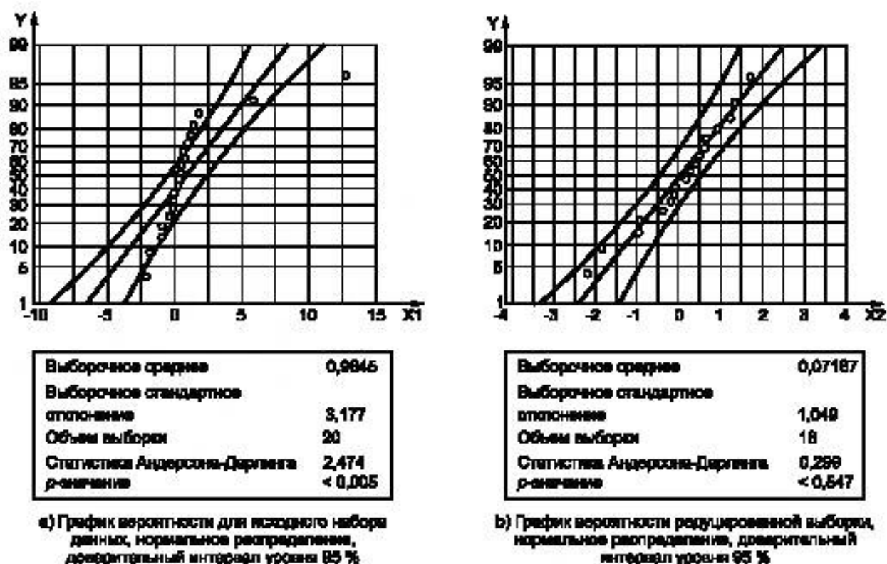
Рисунок 4 — Графики вероятности
