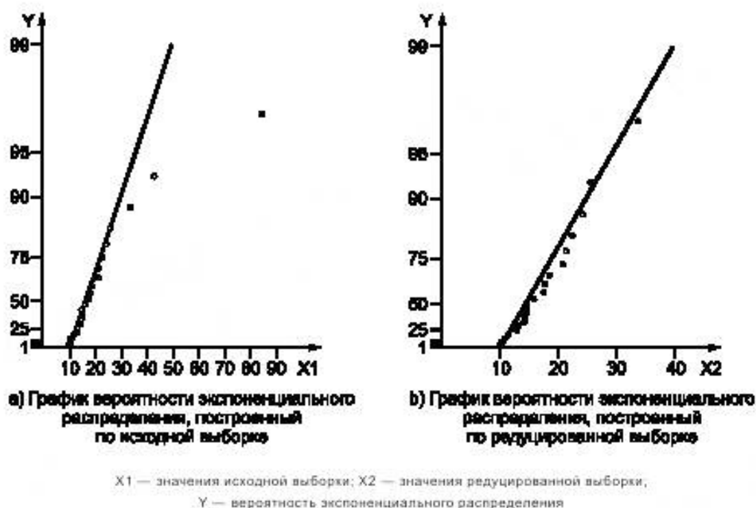
Рисунок 5 — Графики вероятности экспоненциального распределения
