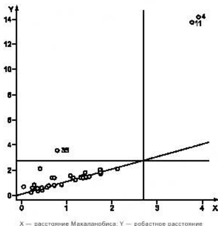
Рисунок 8 — График расстояния Махаланобиса и робастного расстояния
