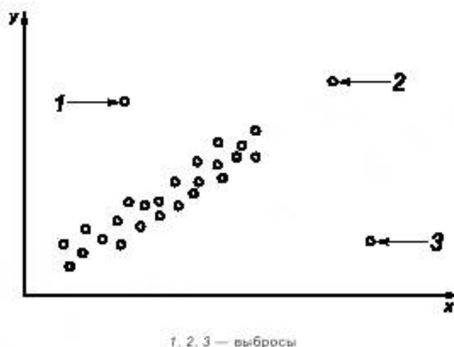
Рисунок 9 — График рассеяния точек (Y,X)
