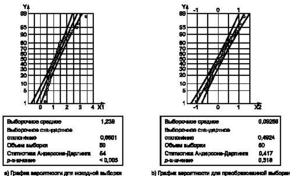
Рисунок 7 — Графики вероятности для исходных и преобразованных данных
