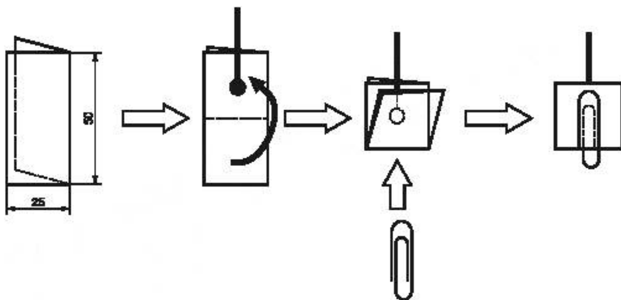
Рисунок 3 — Установка испытуемого образца
