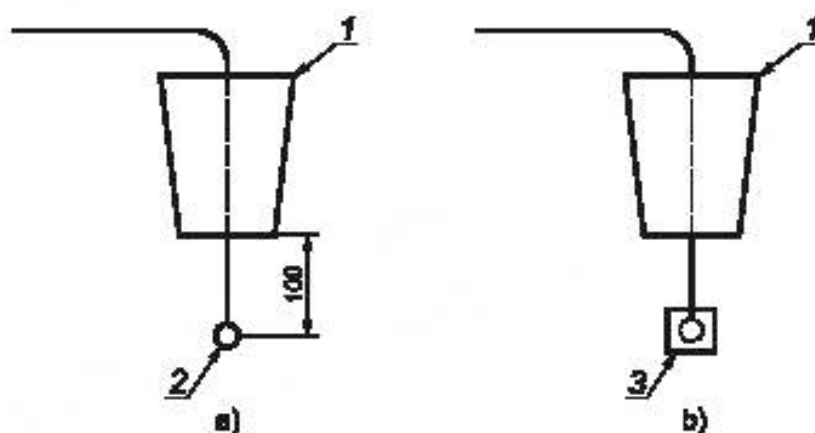
Рисунок 1 — Конфигурация испытательной установки
