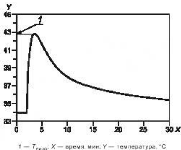
Рисунок 4 — Данные определения гигроскопического и экзотермического свойств
