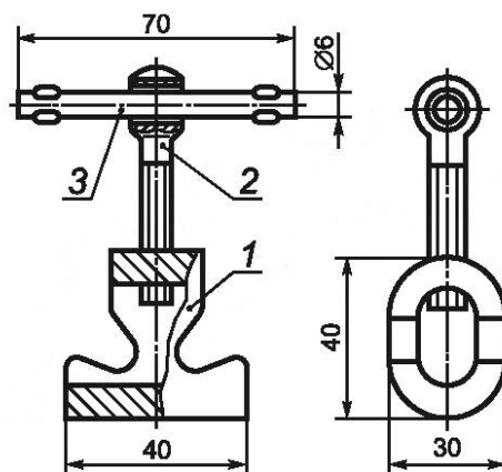
1 — зажим; 2 — болт М8х45 по ГОСТ 3033; 3 — вороток
