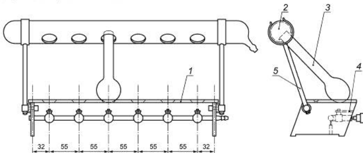
1 — полка из термостойкого теплоизоляционного материала; 2 — выпускная трубка; 3 — колба для кипячения; 4 — микрогорелка; 5 — опорный стержень с регулировкой угла наклона и длины
