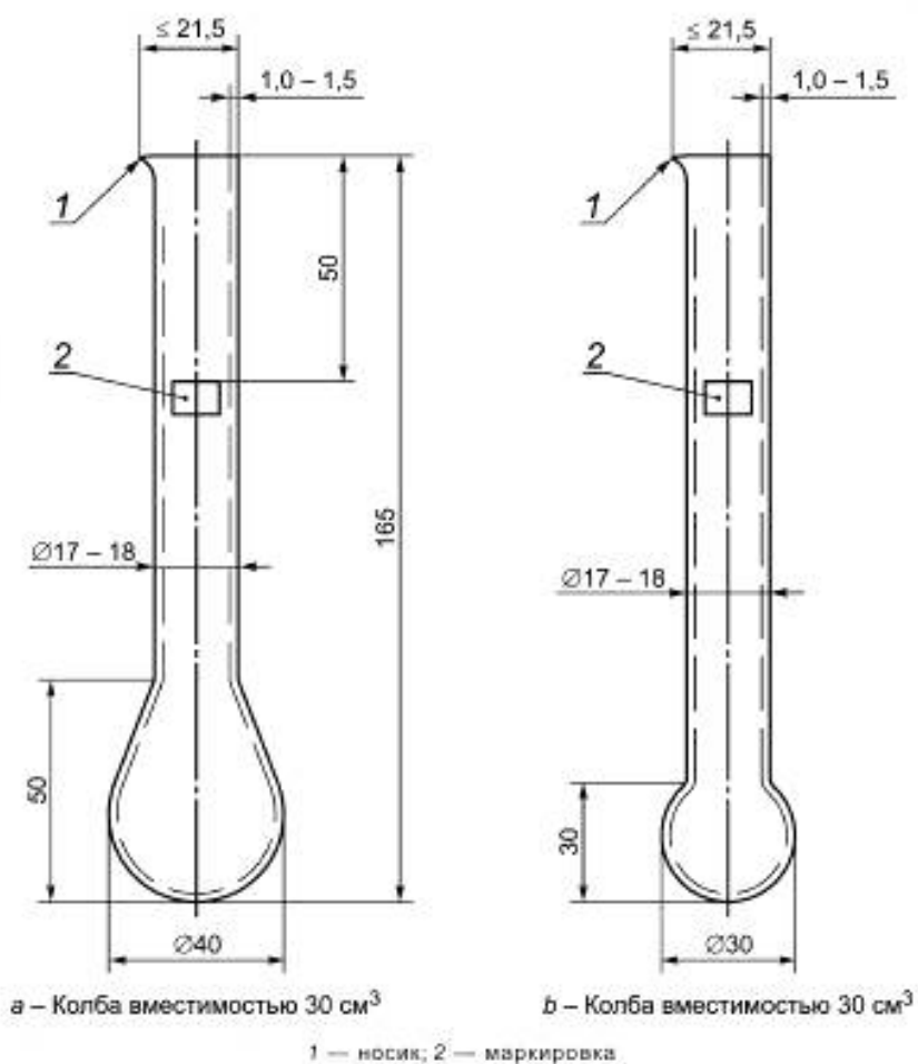
Рисунок 3 — Колбы для кипячения для полумикрометода
