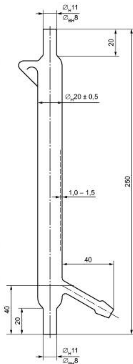
Рисунок 8 — Рубашка холодильника для полумикрометода
