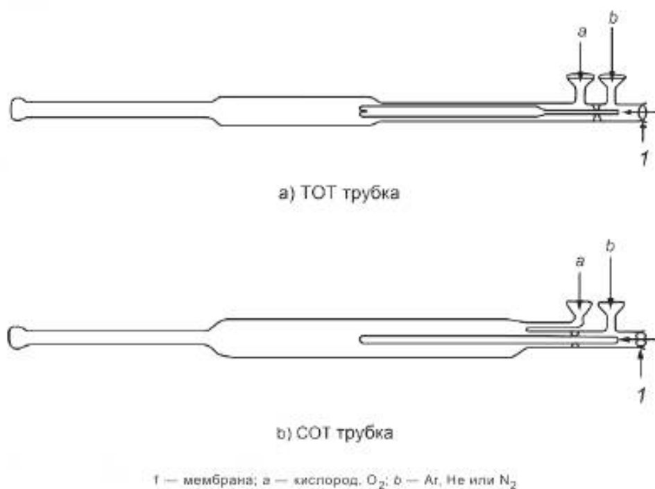
Рисунок 2 — Типовые конструкции трубок для сжигания
