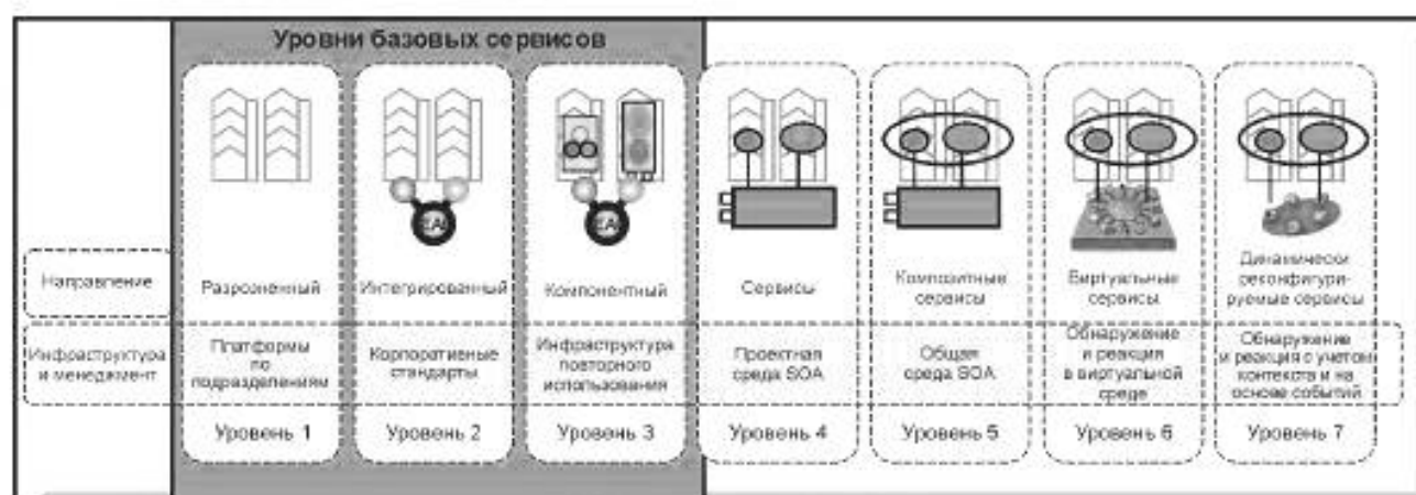
Рисунок 9 — Направление «Инфраструктура и менеджмент» в модели OSIMM
