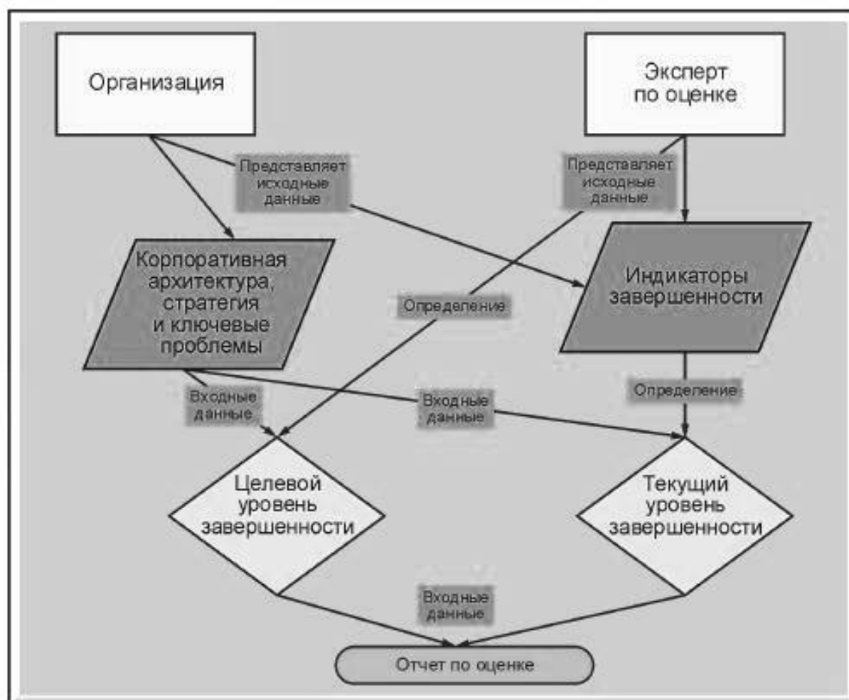
Рисунок 10 — Анализ модели OSIMM
