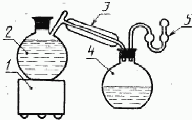
1 — электроплитка; 2 — дистилляционная колба; 3 — холодильник; 4 — колба-приемная; 5 — предохранительная воронка
