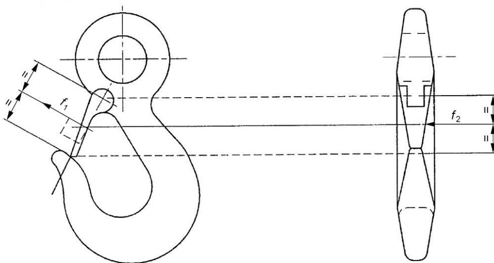
Рисунок 2 — Точки приложения испытательного усилия типа предохранительного замка
