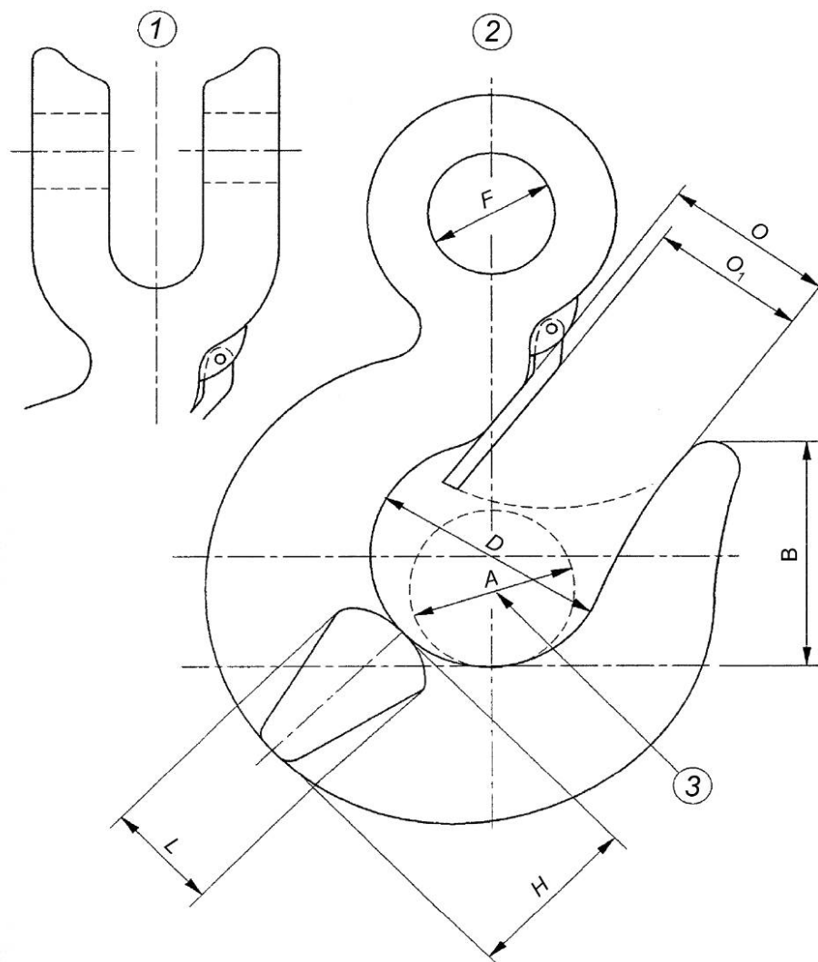
Рисунок 1 — Размеры крюка
