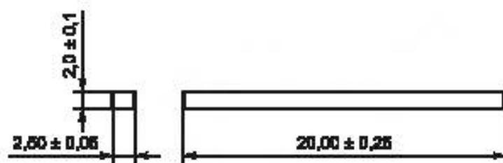
Рисунок 4 — Размеры образца для испытаний
