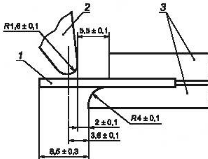
1 — испытываемый образец; 2 — зажимное приспособление; 3 — ударный боек
