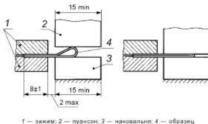
Рисунок 1 — Схема прибора для определения температуры хрупкости
