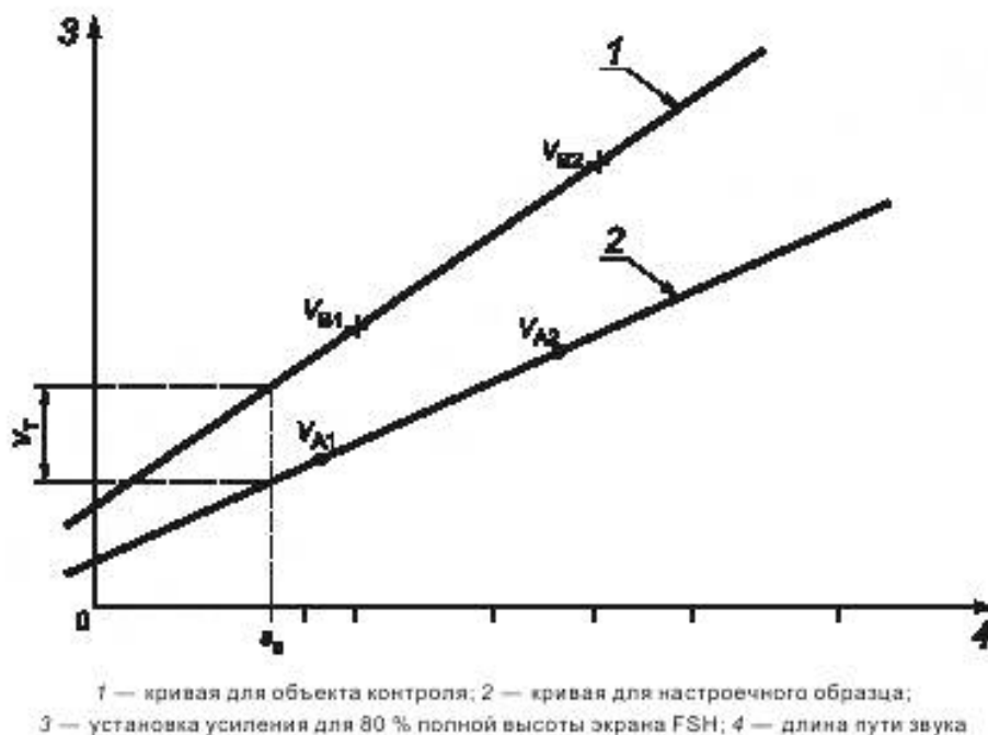
Рисунок 13 — Определение коррекции усиления при использовании сравнительного способа
