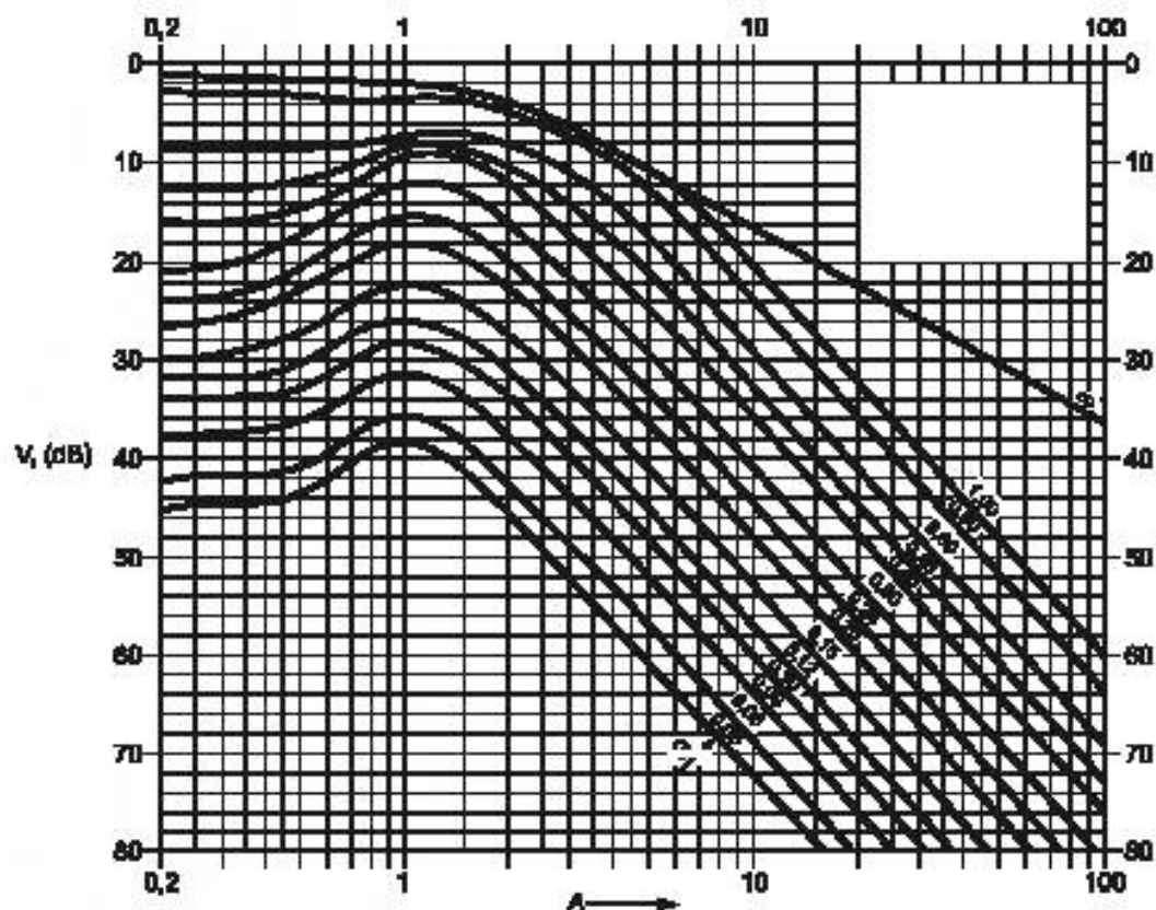
Рисунок 10 — Общая DGS-диаграмма
