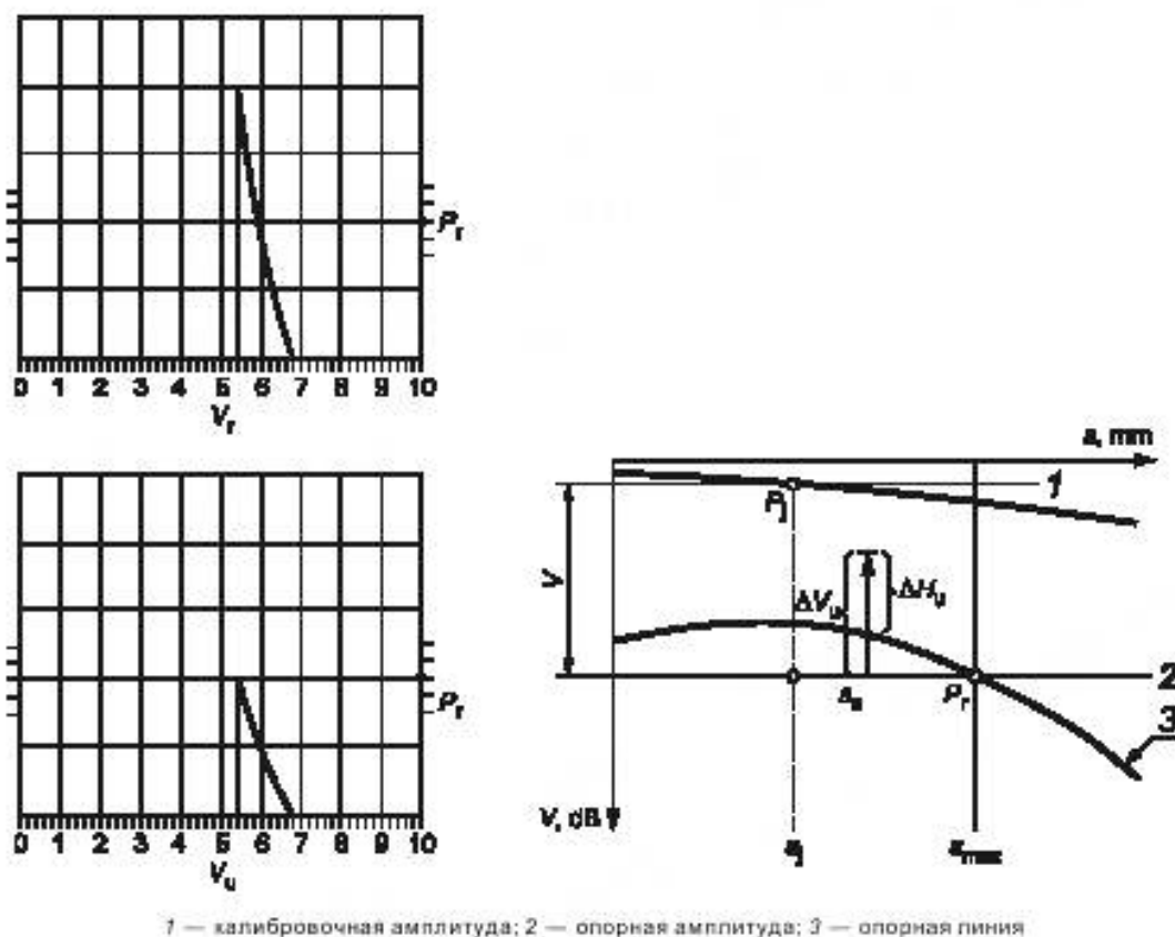
Рисунок 12 — Пример оценки амплитуды эхо-сигнала с использованием способа опорной амплитуды
