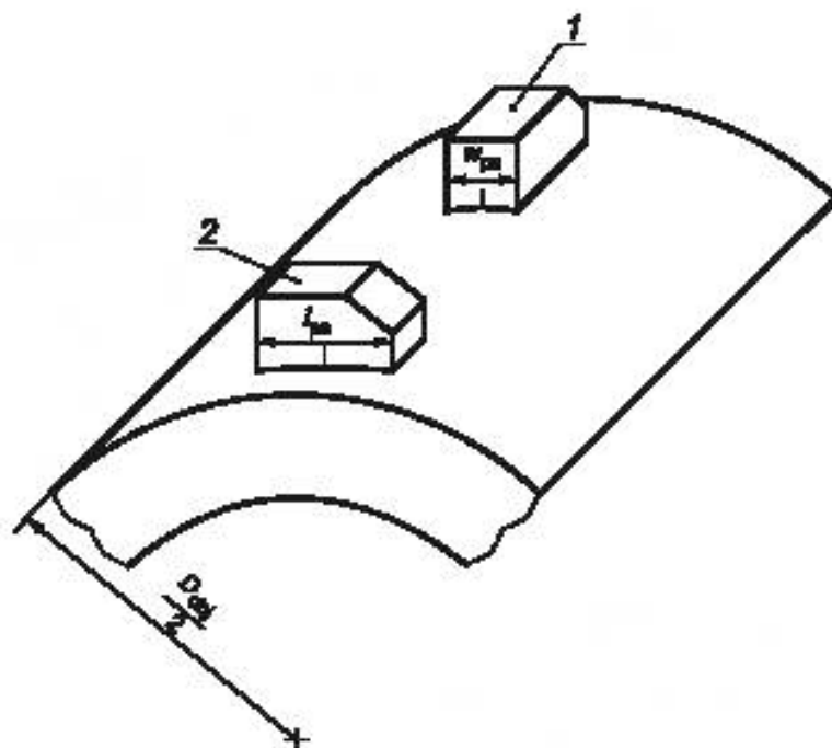
1 — преобразователь, профилированный в поперечном направлении; 2 — преобразователь, профилированный в продольном направлении
