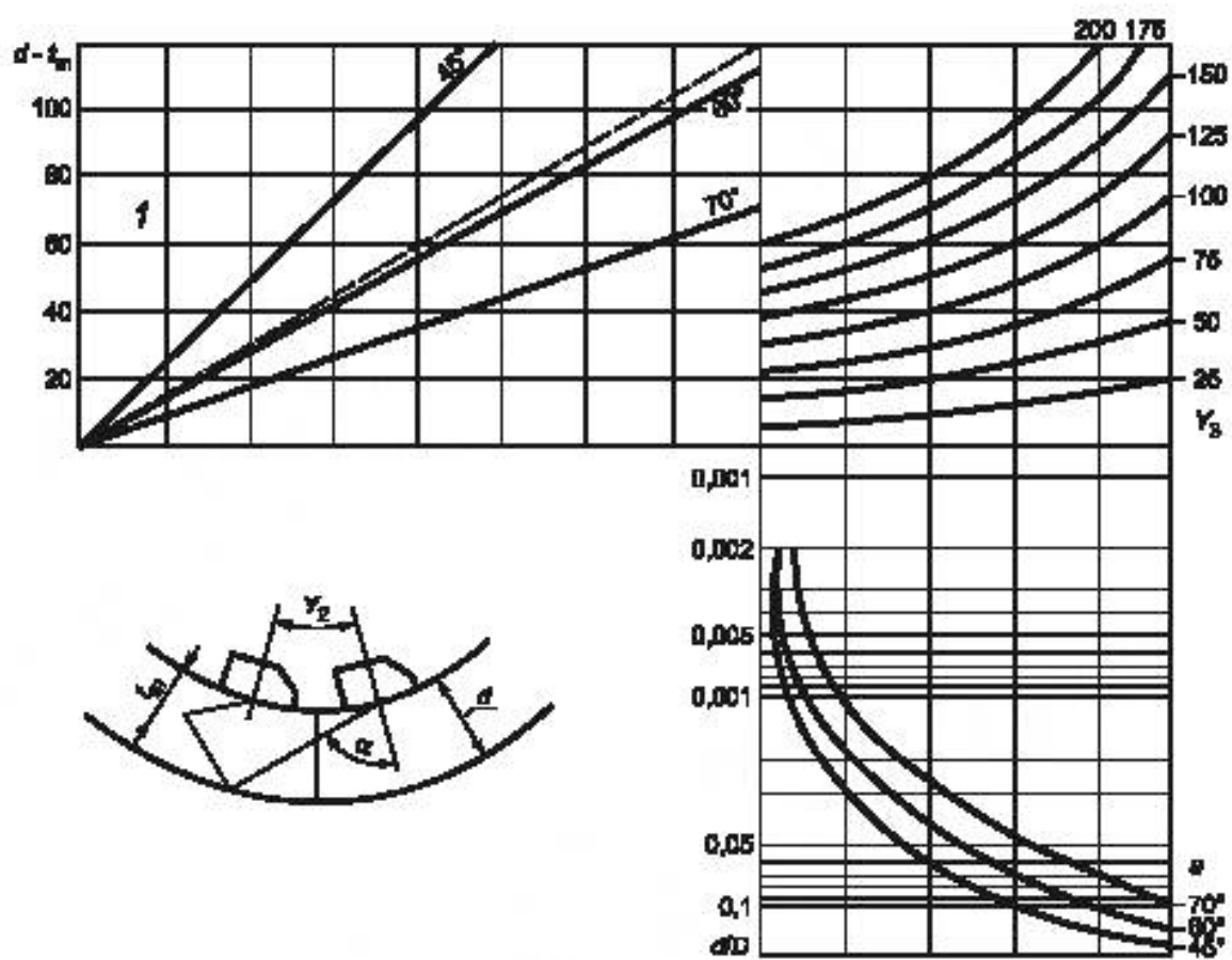
Рисунок А.2 — Номограмма для вогнутых поверхностей
