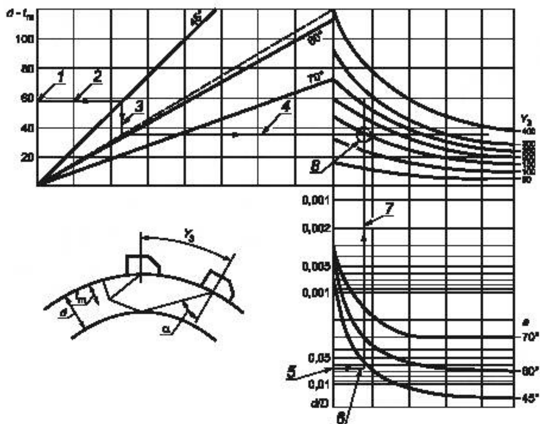
Рисунок А.1 — Номограмма для выпуклых поверхностей
