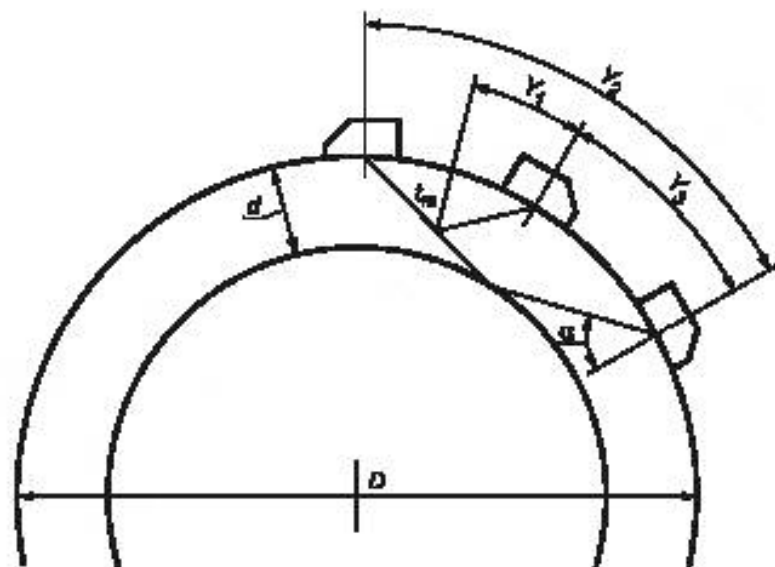
Рисунок 5 — Выпуклая поверхность сканирования
