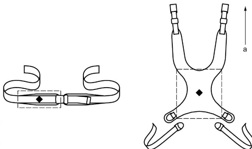
Рисунок 4 — Примеры расположения источников тепла для PSD небольшого размера
