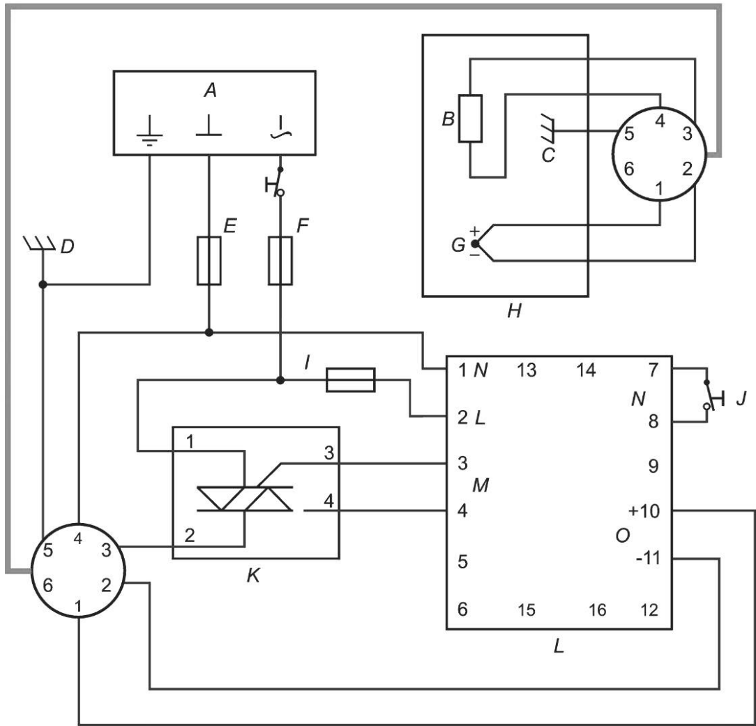
A — питание от сети 230 В переменного тока; B — нагревательный провод; C — заземление; D — заземлительная коробка; E — предохранитель F630 мА; F — предохранитель F630 мА; G — термопара типа K (NiCrNi); H — нагревательный картридж HotSet HotRod 8×80 200 Вт; I — предохранитель 200 мА; J — пусковой переключатель; K — твердотельное реле croud D2425; L — терморегулятор HotSet HotControl C248; M — dou2; N — цифровой вход; O — термомолния
