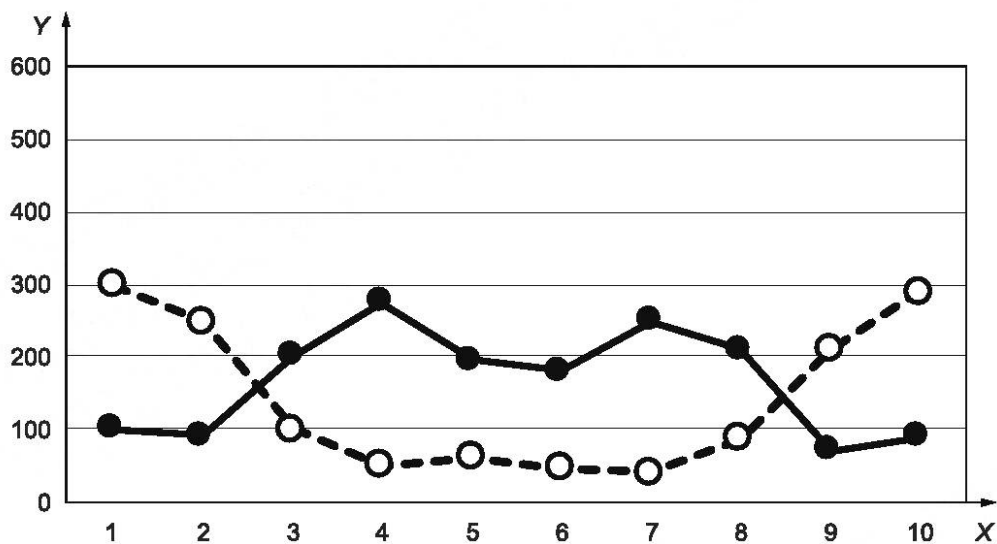
Рисунок 9 — Пример сравнительного линейного графика показаний давления от осевой линии датчиков для двух разных подушек
