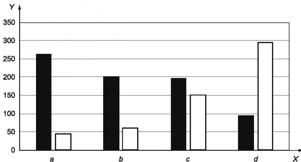
Рисунок 10 — Пример сравнительной гистограммы среднего давления по высоте для двух разных подушек
