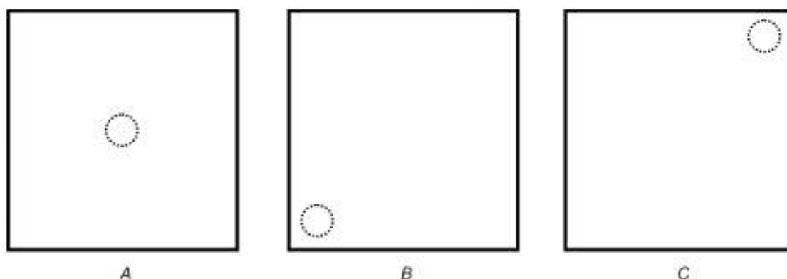
а) Зона удара при испытании деревянным снарядом (для каждого типа остекления)
