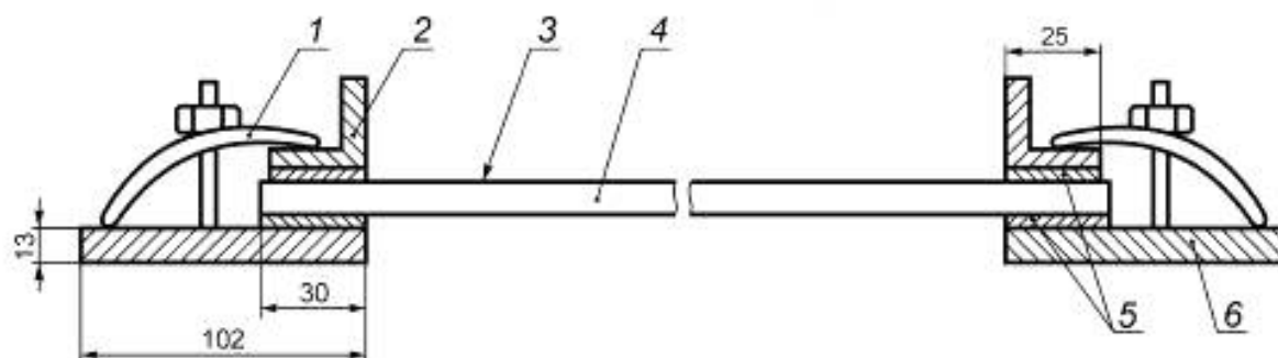
1 — зажим; 2 — внутренняя рама; 3 — поверхность остекления 900 × 1100 мм; 4 — образец; 5 — резина; 6 — наружная рама
