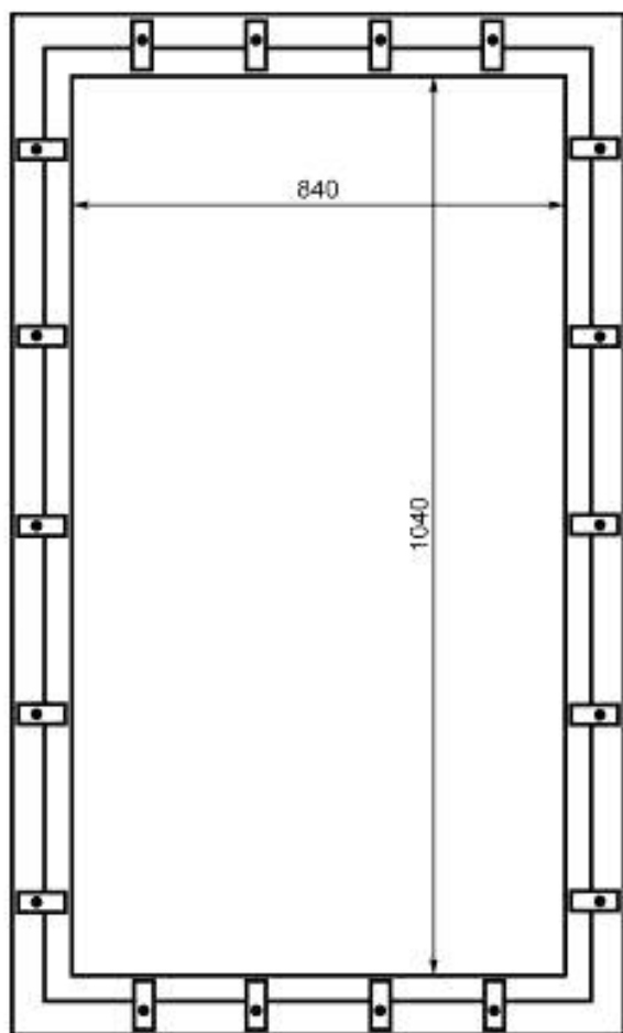
Рисунок В.2 — Наружная рама
