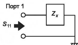
Рисунок 12 — Однопортовое измерение двухвыводного оборудования
