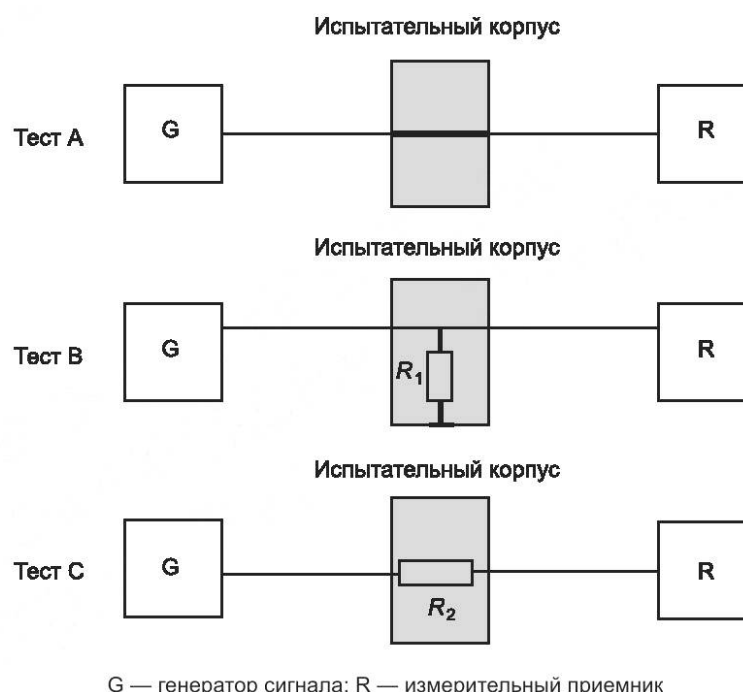
Рисунок 10 — Схема испытаний для проверки измерительной схемы без смещения
