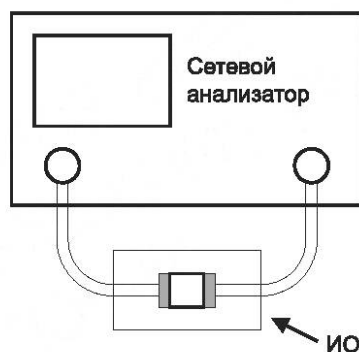
Рисунок 15 — Схема измерения S-параметров двух портов
