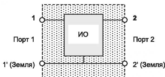
Рисунок 2 — Измерительная схема S-параметров оборудования с тремя выводами
