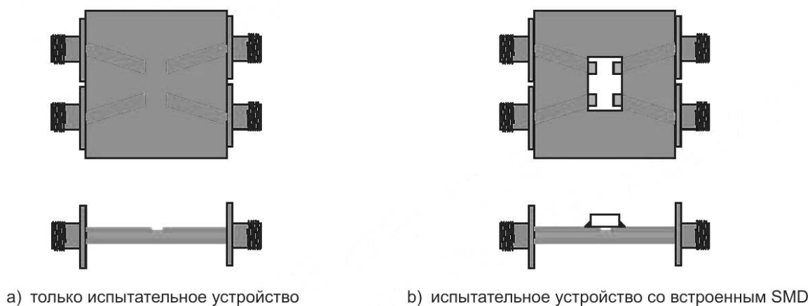
Рисунок G.9 — Испытательное устройство для S-параметров четырех портов SMD
