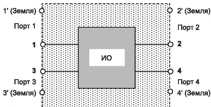
Рисунок 3 — Измерительная схема S-параметров оборудования с четырьмя портами
