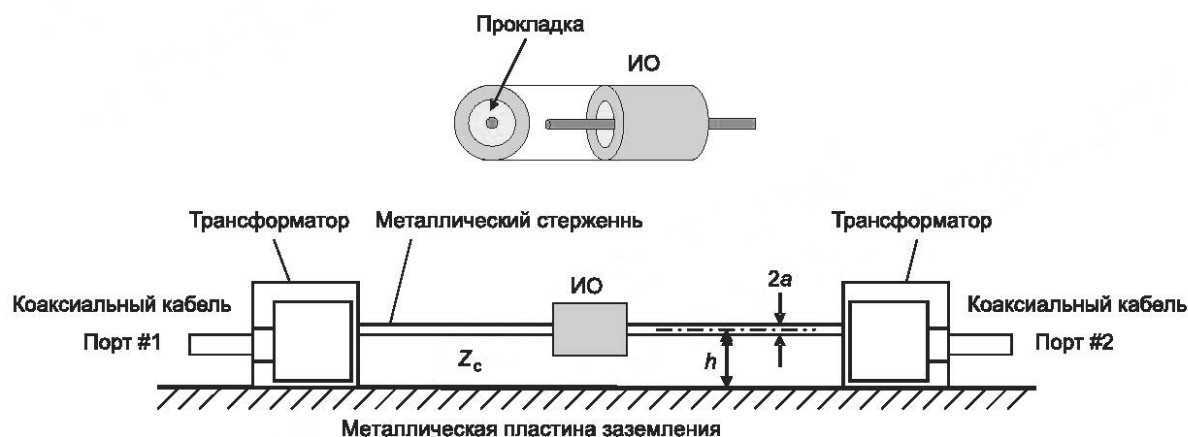
Рисунок Н.1 — Измерение S-параметров ИО без выводов
