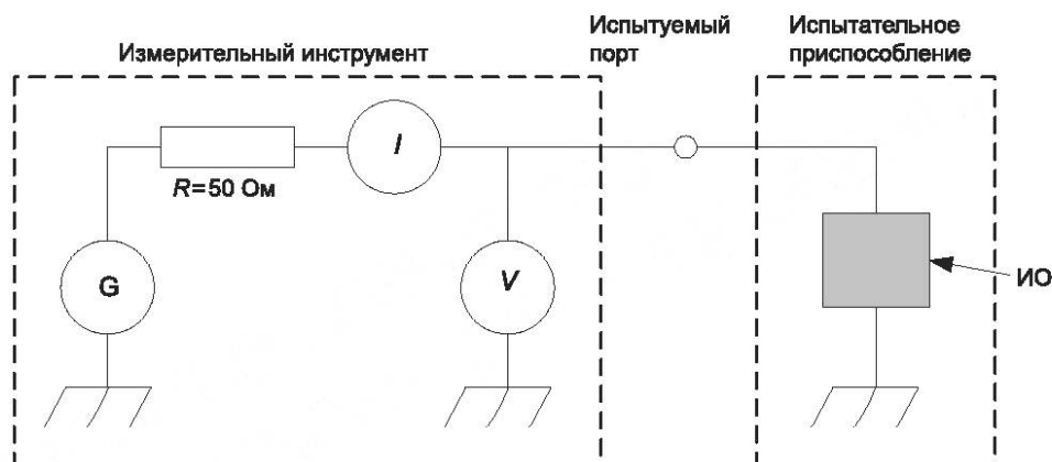
Рисунок F.3 — Схема измерений для SMD
