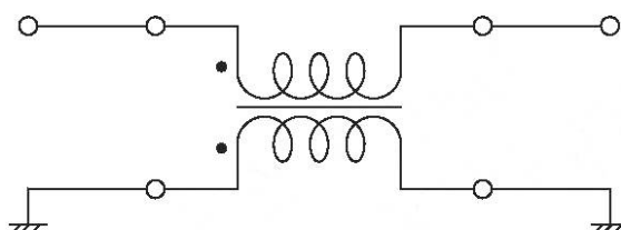
Рисунок G.5 — Схема измерений характеристик в дифференциальном режиме
