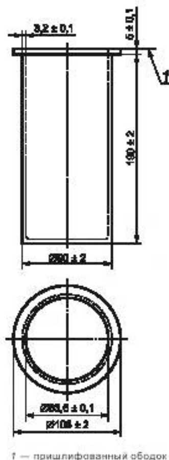
Рисунок 1 — Химический стакан
