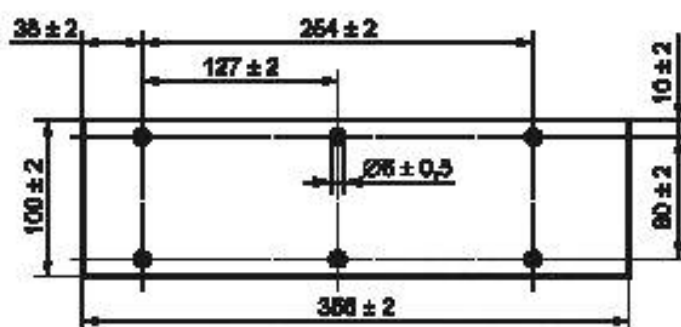
Рисунок 1 — Образец для испытаний
