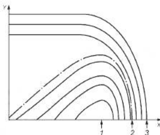
Рисунок H.3 — Пример дебита относительно давления через устройство для регулирования дебита
