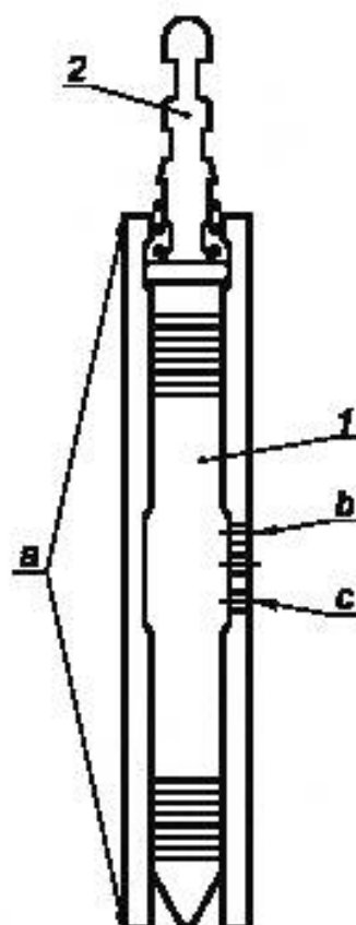
Рисунок О.1 — Схема испытательной установки измерения расхода
