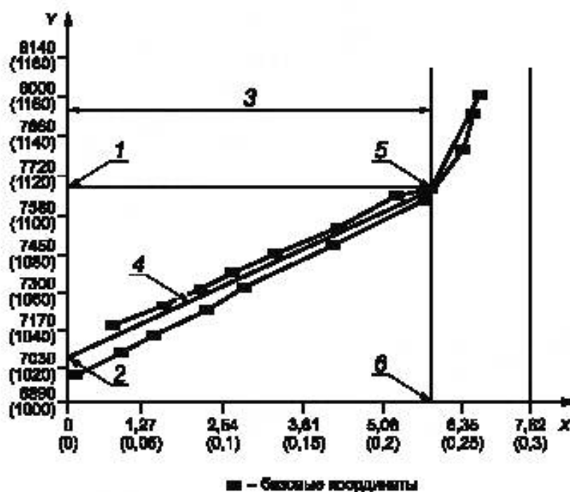
Рисунок G.4 — Пример нанесения данных перемещения штанги
