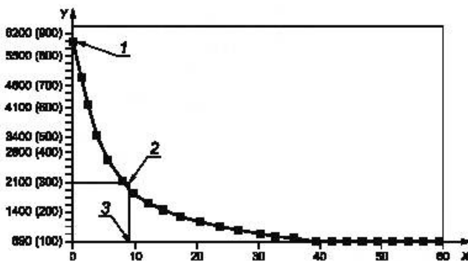
Рисунок Н.8 — Пример срабатывания испытательной установки
