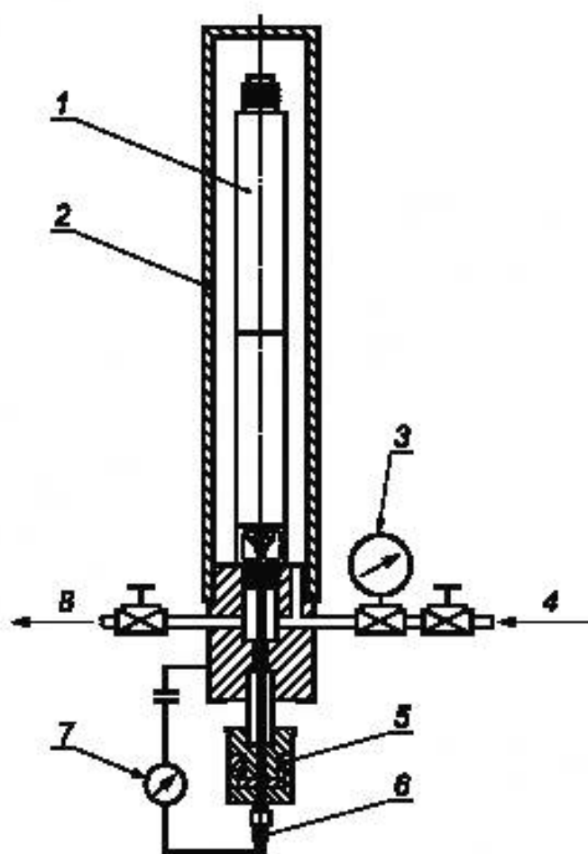
1 — устройство для регулирования дебита; 2 — испытательная установка; 3 — манометр; 4 — прибор для контроля газа; 5 — изолирующая втулка; 6 — микрометр; 7 — омметр; 8 — выделение газа
