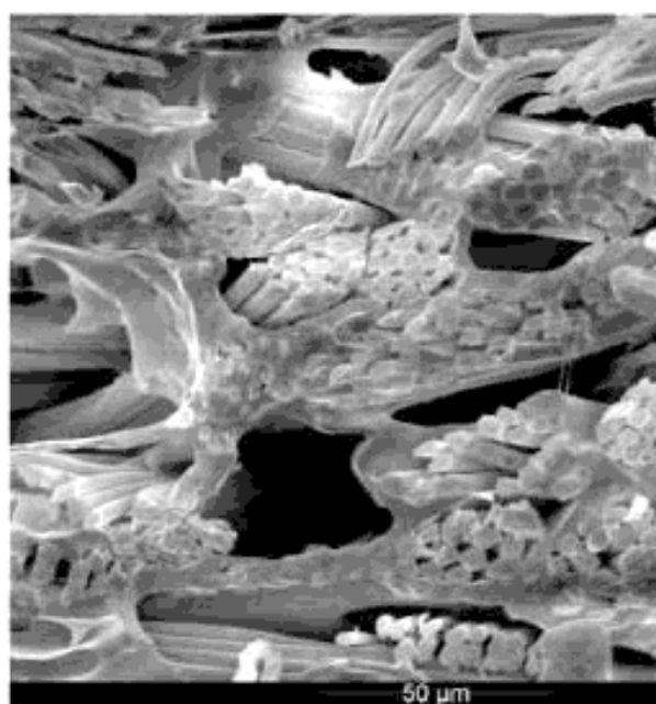
б) Сечение материала микрофибра при большом увеличении
