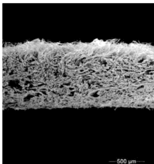
а) Сечение материала микрофибра при небольшом увеличении
