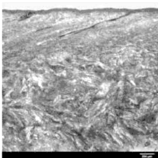
Рисунок В.1 — Типичное сечение кожи, выработанной из шкуры крупного рогатого скота (далее — КРС), с облагороженной лицевой поверхностью и толщиной покрытия менее 150 мкм
