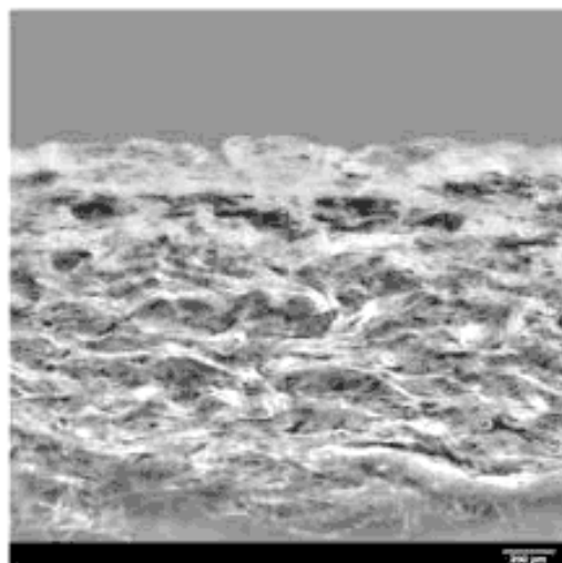
Рисунок В.2 — Типичное сечение шеврета
