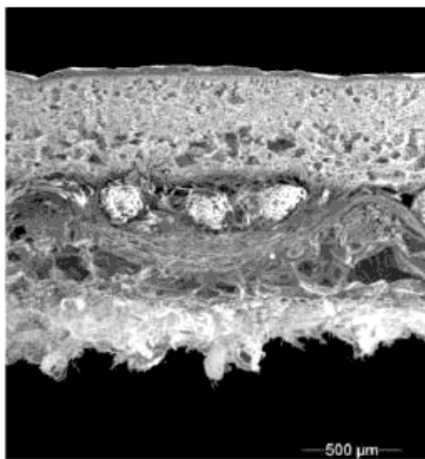
Рисунок А.12 — Сечение полимерного материала, дублированного с кожными волокнами
