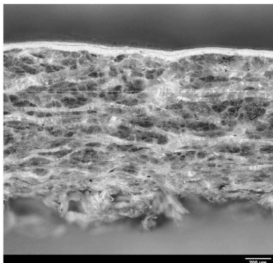
Рисунок В.5 — Типичное сечение из спилка с покрытием, выработанного из кожи КРС
