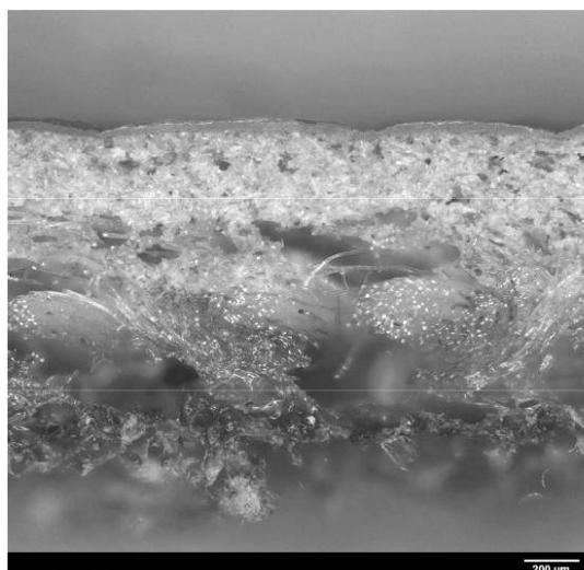
Рисунок В.12 — Синтетический материал с дублированными кожевенными волокнами
