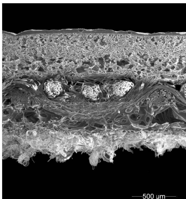
Рисунок А.12 — Сечение полимерного материала, дублированного с коженными волокнами
