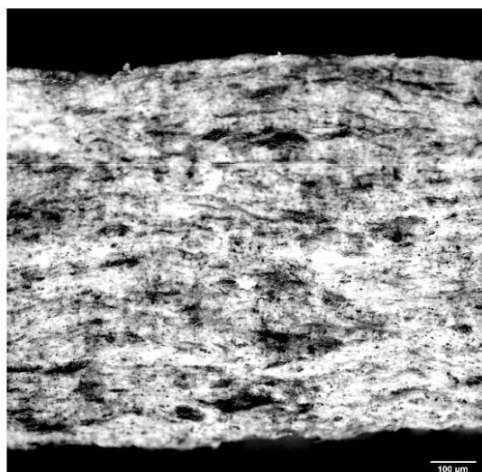
Рисунок В.10 — Типичное сечение листового материала, выработанного из кожевенных волокон
