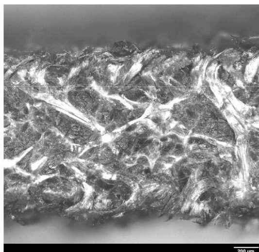
Рисунок В.6 — Типичное сечение велюра, выработанного из кожи КРС
