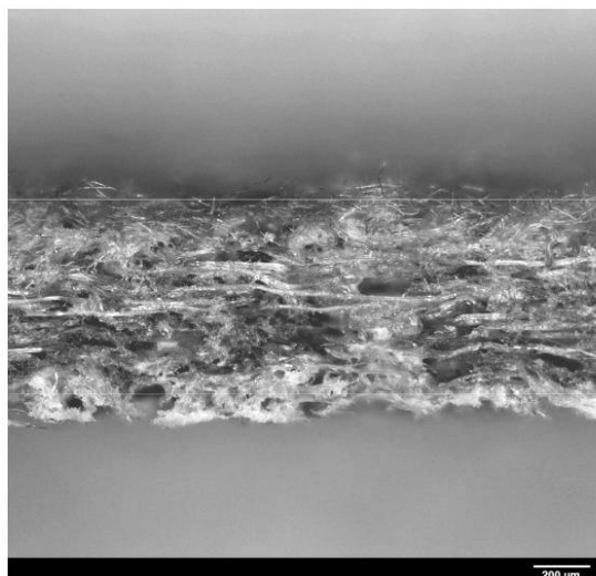
Рисунок В.7 — Типичное сечение материала микрофибра
