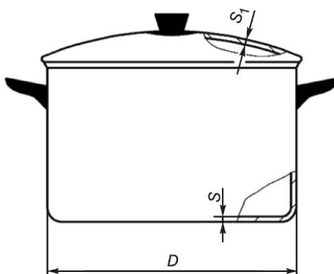
Рисунок 1 — Кастрюля цилиндрическая
