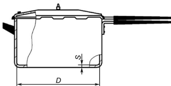
Рисунок 12 — Кастрюля-сковарка
