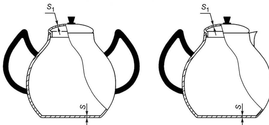
Рисунок 52 — Молочник (сахарница)
