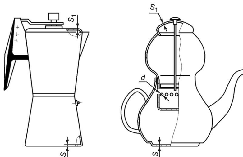
Рисунок 30 — Кофеварка комбинированная
