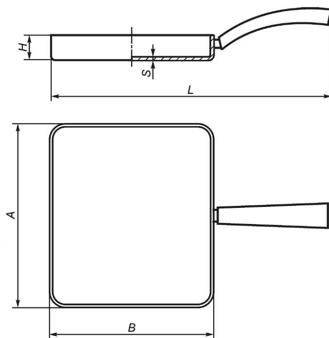
Рисунок 15 — Сковорода прямоугольная
