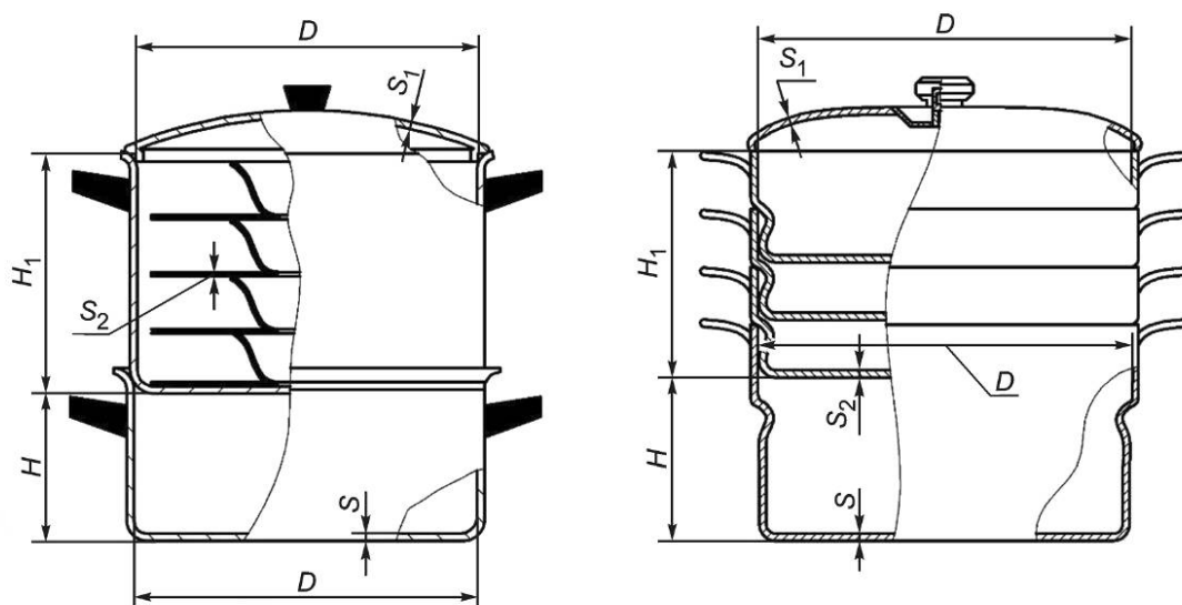
Рисунок 25 — Мантоварка
