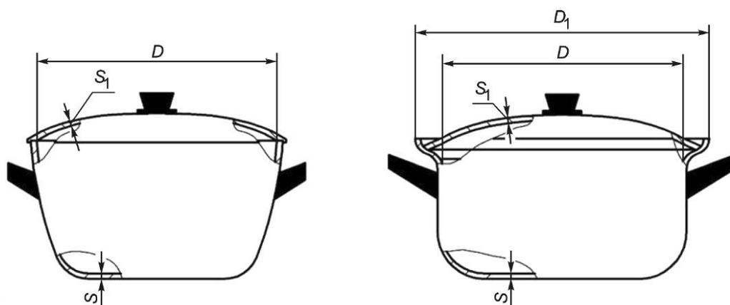
Рисунок 3 — Кастрюля полусферическая
