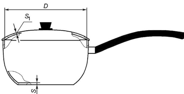
Рисунок 2 — Кастрюля сферическая
