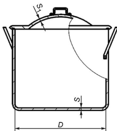
Рисунок 31 — Котел
