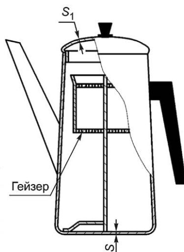
Рисунок 28 — Кофейник
