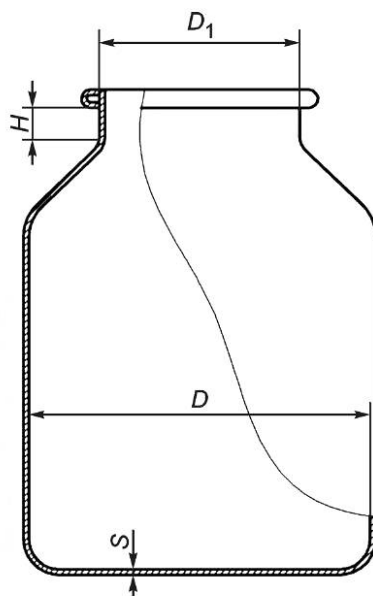
Рисунок 54 — Бидон специальный
