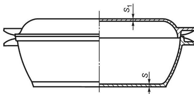
Рисунок 19 — Утятница и гусятница
