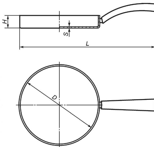
Рисунок 18 — Сотейник
