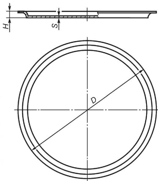
Рисунок 50 — Поднос круглый
