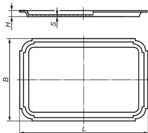
Рисунок 51 — Поднос прямоугольный
