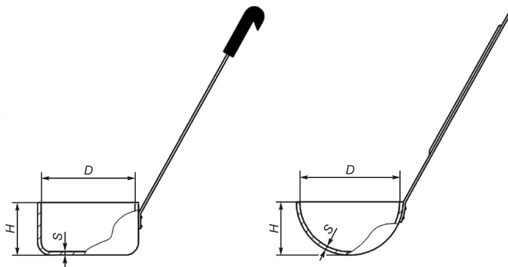
Рисунок 42 — Ложка разливательная
