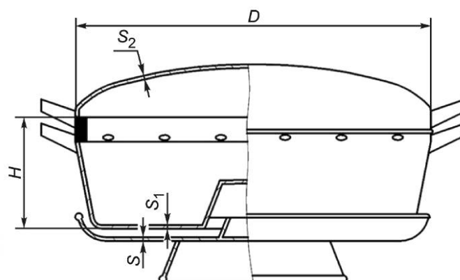
Рисунок 26 — Печь «Чудо»
