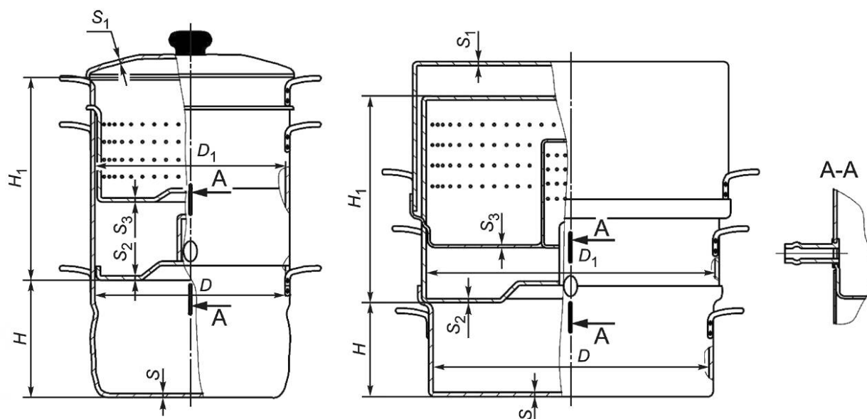
Рисунок 24 — Соковарка
