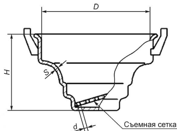
Рисунок 41 — Цедилка для молока
