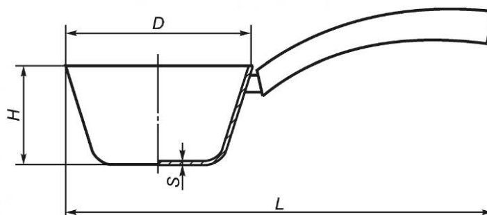
Рисунок 20 — Ковш
