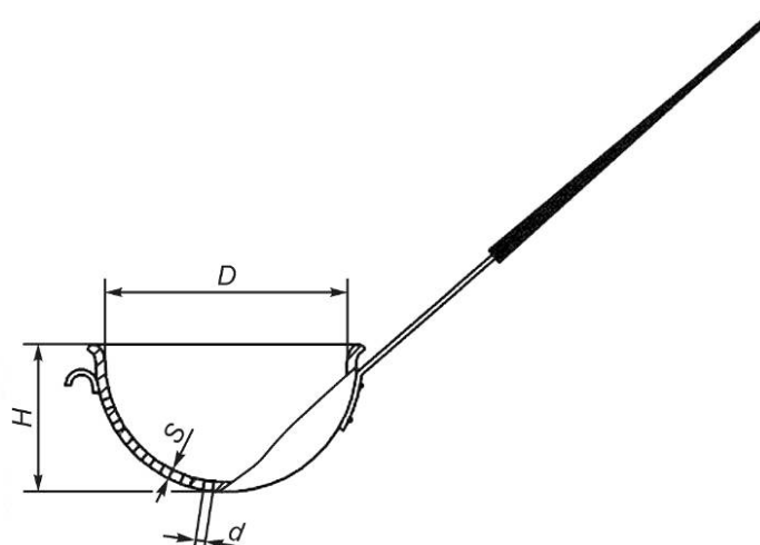
Рисунок 40 — Цедилка
