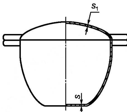
Рисунок 21 — Казан
