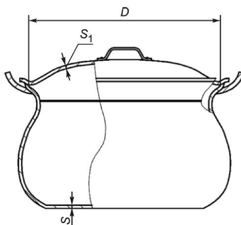
Рисунок 6 — Кастрюля выпуклая
