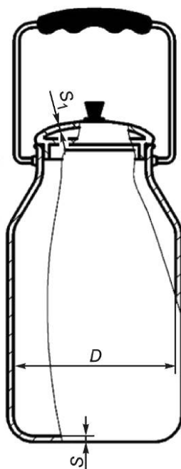
Рисунок 32 — Бидон
