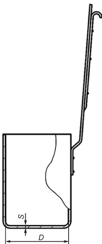
Рисунок 39 — Кружка разливательная
