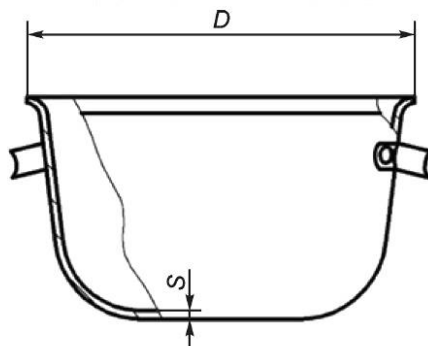
Рисунок 23 — Казанок
