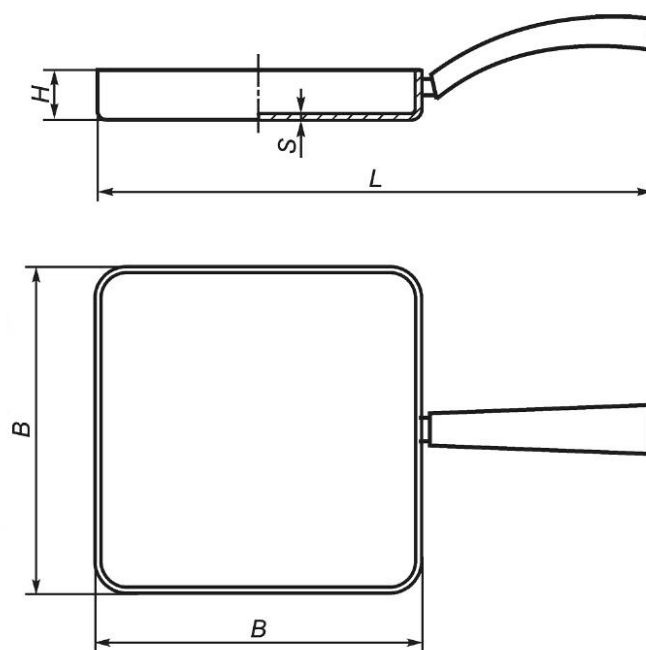
Рисунок 16 — Сковорода квадратная
