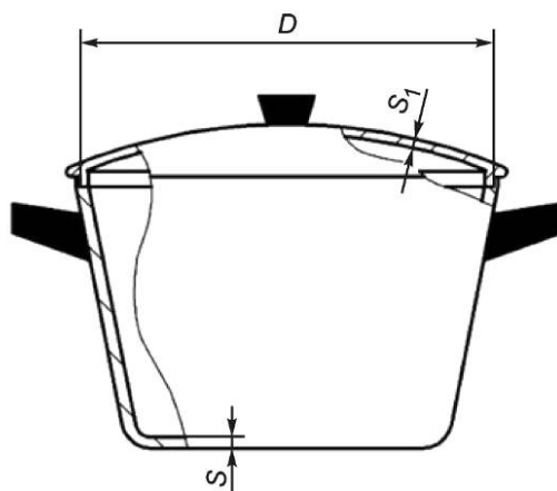
Рисунок 4 — Кастрюля коническая
