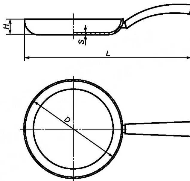
Рисунок 13 — Сковорода
