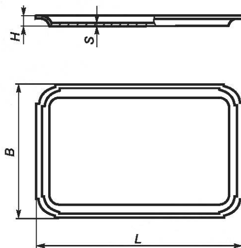
Рисунок 51 — Поднос прямоугольный
