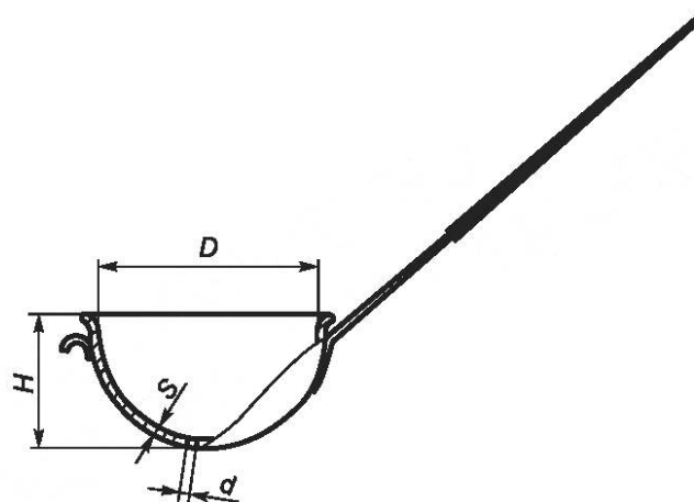
Рисунок 40 — Цедилка
