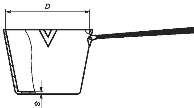
Рисунок 5 — Кастрюля коническая со сливом
