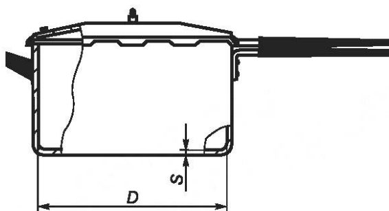
Рисунок 12 — Кастрюля-сковарка
