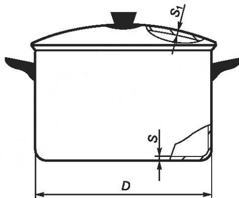
Рисунок 1 — Кастрюля цилиндрическая
