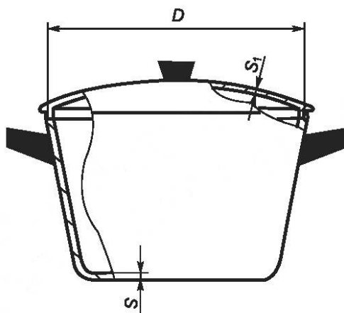
Рисунок 4 — Кастрюля коническая
