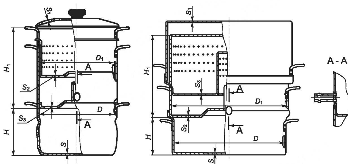
Рисунок 24 — Соковарка
