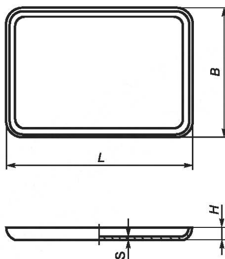
Рисунок 49 — Противень
