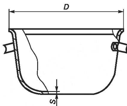
Рисунок 23 — Казанок
