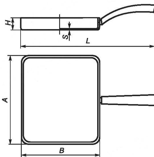
Рисунок 15 — Сковорода прямоугольная
