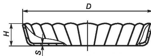
Рисунок 48 — Форма для выпечки
