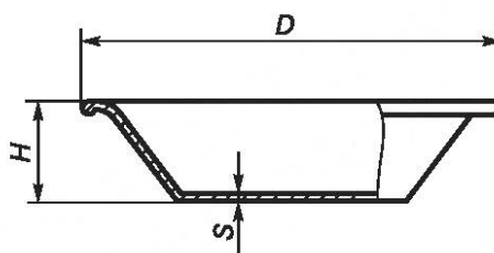
Рисунок 37 — Тарелка
