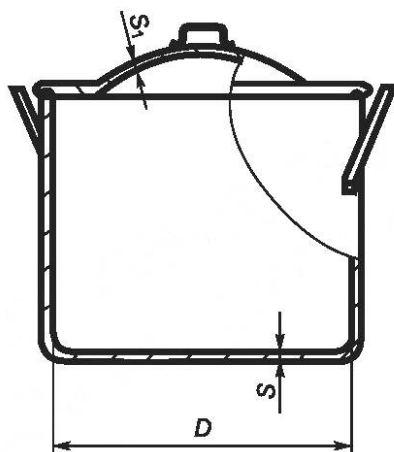
Рисунок 31 — Котел
