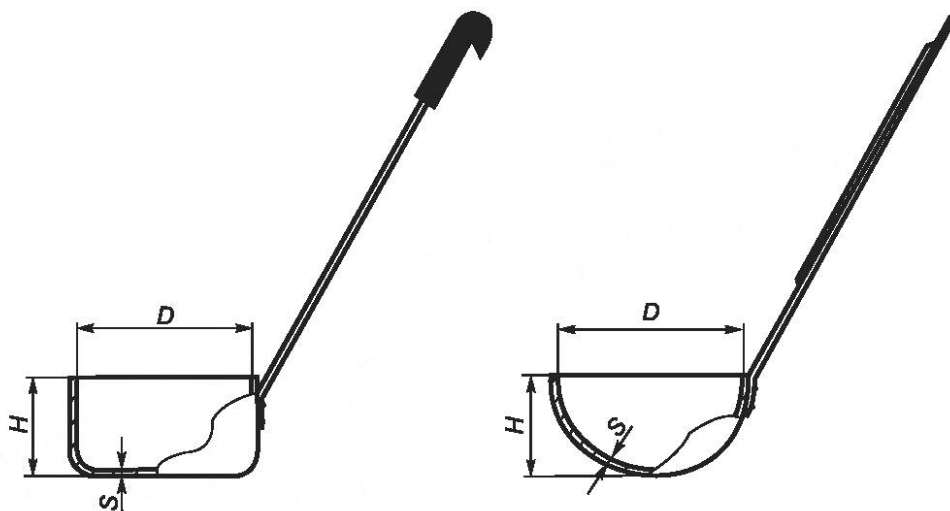
Рисунок 42 — Ложка разливательная
