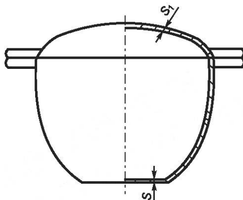
Рисунок 21 — Казан
