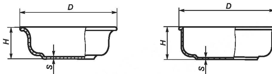
Рисунок 36 — Миска
