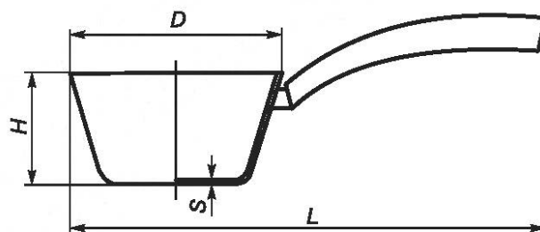
Рисунок 20 — Ковш
