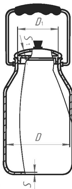
Рисунок 32 — Бидон
