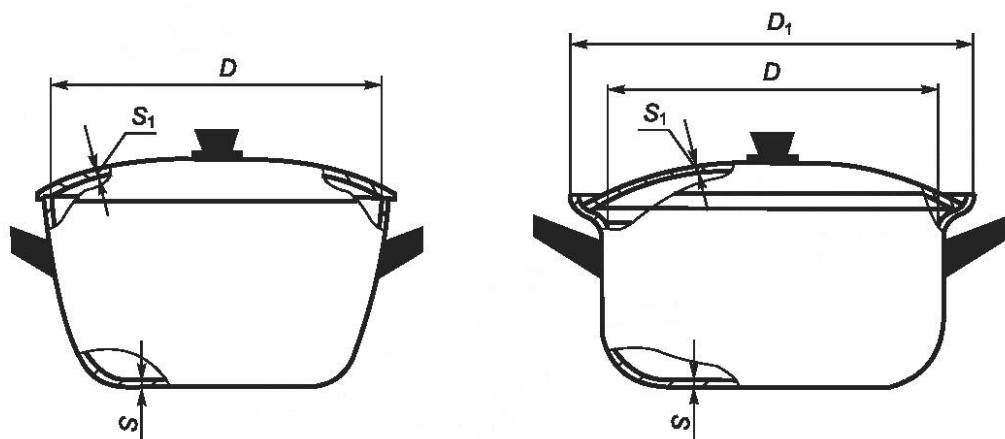
Рисунок 3 — Кастрюля полусферическая
