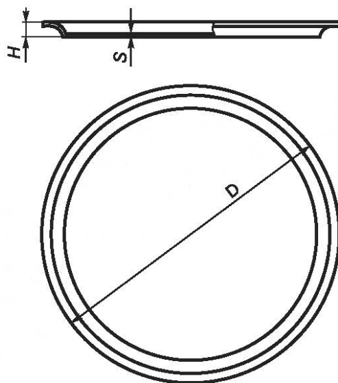
Рисунок 50 — Поднос круглый
