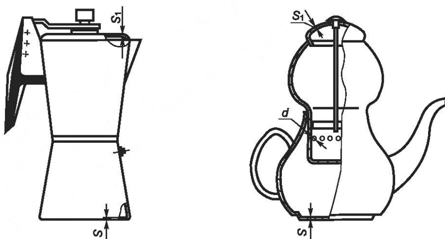
Рисунок 30 — Кофеварка комбинированная
