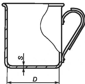
Рисунок 38 — Кружка
