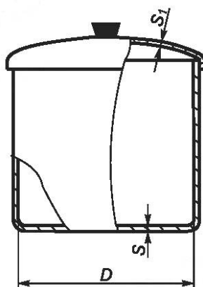
Рисунок 45 — Банка круглая для хранения сыпучих продуктов
