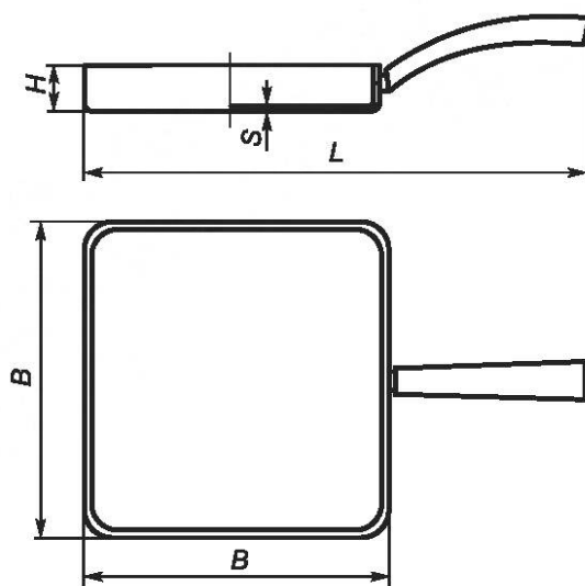
Рисунок 16 — Сковорода квадратная
