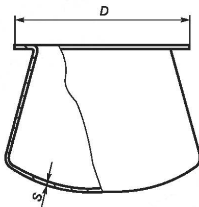
Рисунок 22 — Казан конический
