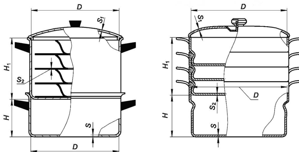
Рисунок 25 — Мантоварка
