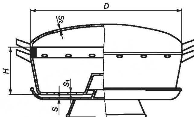
Рисунок 26 — Печь «Чудо»
