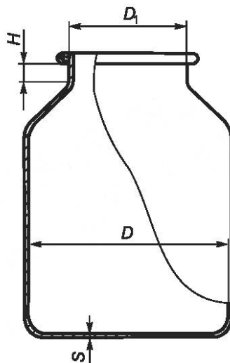
Рисунок 54 — Бидон специальный
