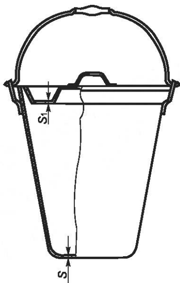
Рисунок 34 — Ведро
