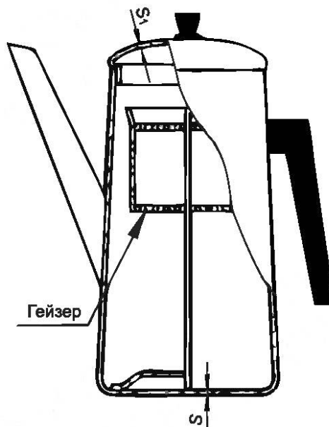
Рисунок 28 — Кофейник
