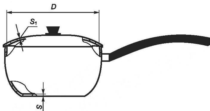
Рисунок 2 — Кастрюля сферическая
