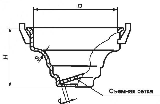
Рисунок 41 — Цедилка для молока
