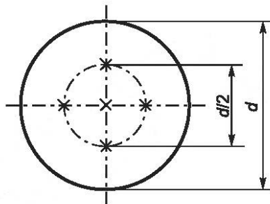
Рисунок 55 — Схема размещения материалов при проведении испытания на сохранность формы изделия с плакирующим покрытием
