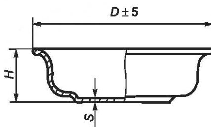
Рисунок 35 — Таз
