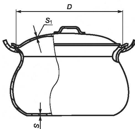
Рисунок 6 — Кастрюля выпуклая
