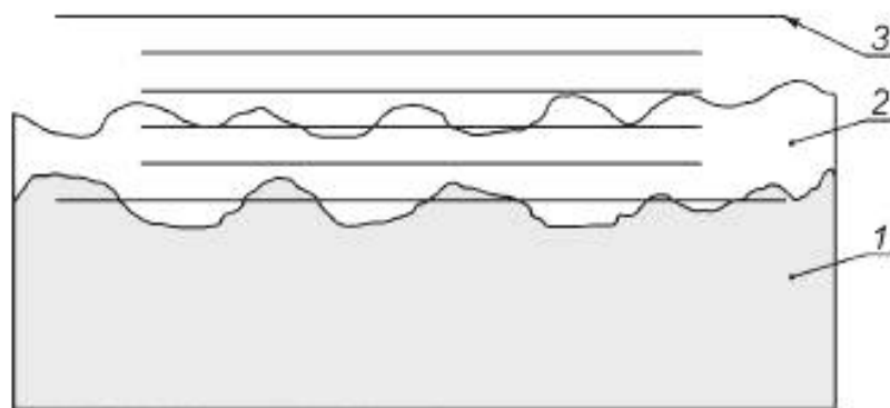
1 — кожа; 2 — покрытие; 3 — градуированная шкала параллельных линий
