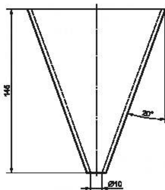
Рисунок 1 — Определение скорости растекания с помощью воронки
