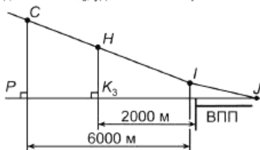
Рисунок 3 — Типичная траектория снижения на посадку
