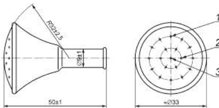
1 — 12 отверстий диаметром (0,9 \pm 0,05) мм на окружности диаметром (21,4 \pm 0,05) мм; 2 — 6 отверстий диаметром (0,9 \pm 0,05) мм на окружности диаметром (10 \pm 0,05) мм; 3 — 1 отверстие диаметром (0,9 \pm 0,05) мм в центре
