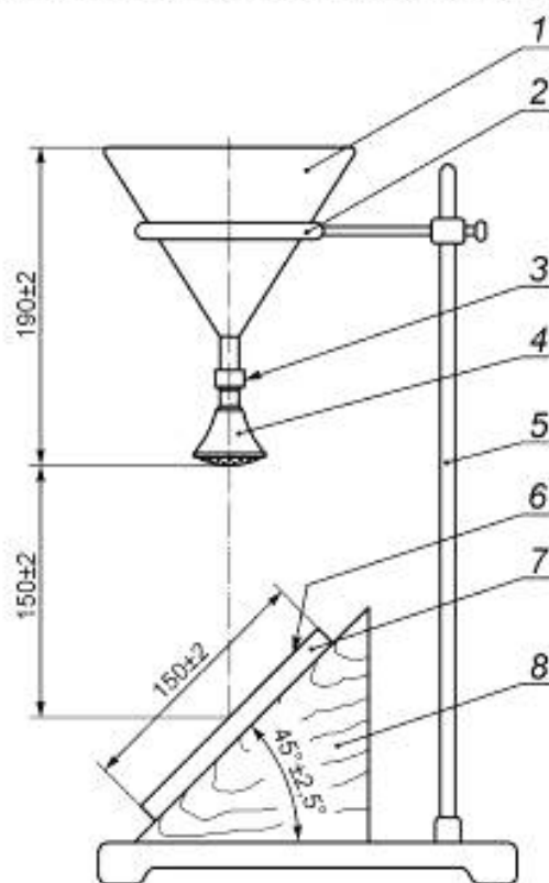
1 — стеклянная воронка диаметром (150 \pm 2) мм; 2 — кольцевой кронштейн; 3 — резиновая трубка; 4 — разбрызгивающее сопло; 5 — штатив; 6 — образец; 7 — держатель образца; 8 — подставка (например, дерево)
