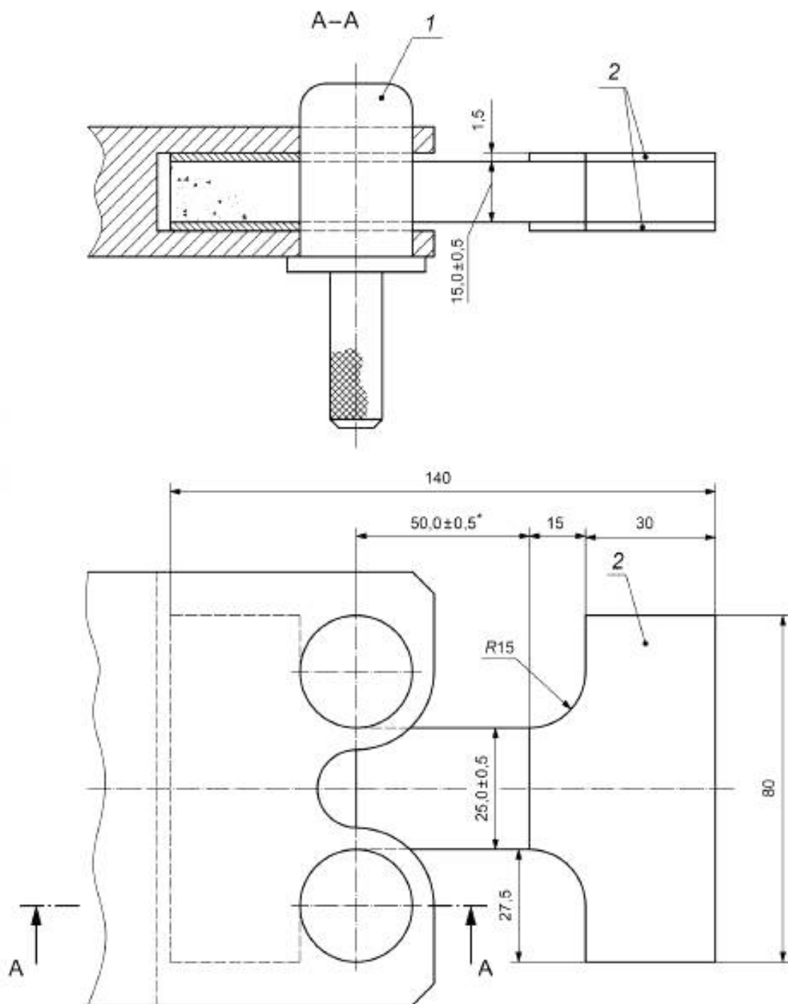
Рисунок 3 — Образец типа 3 с металлическими пластинами
