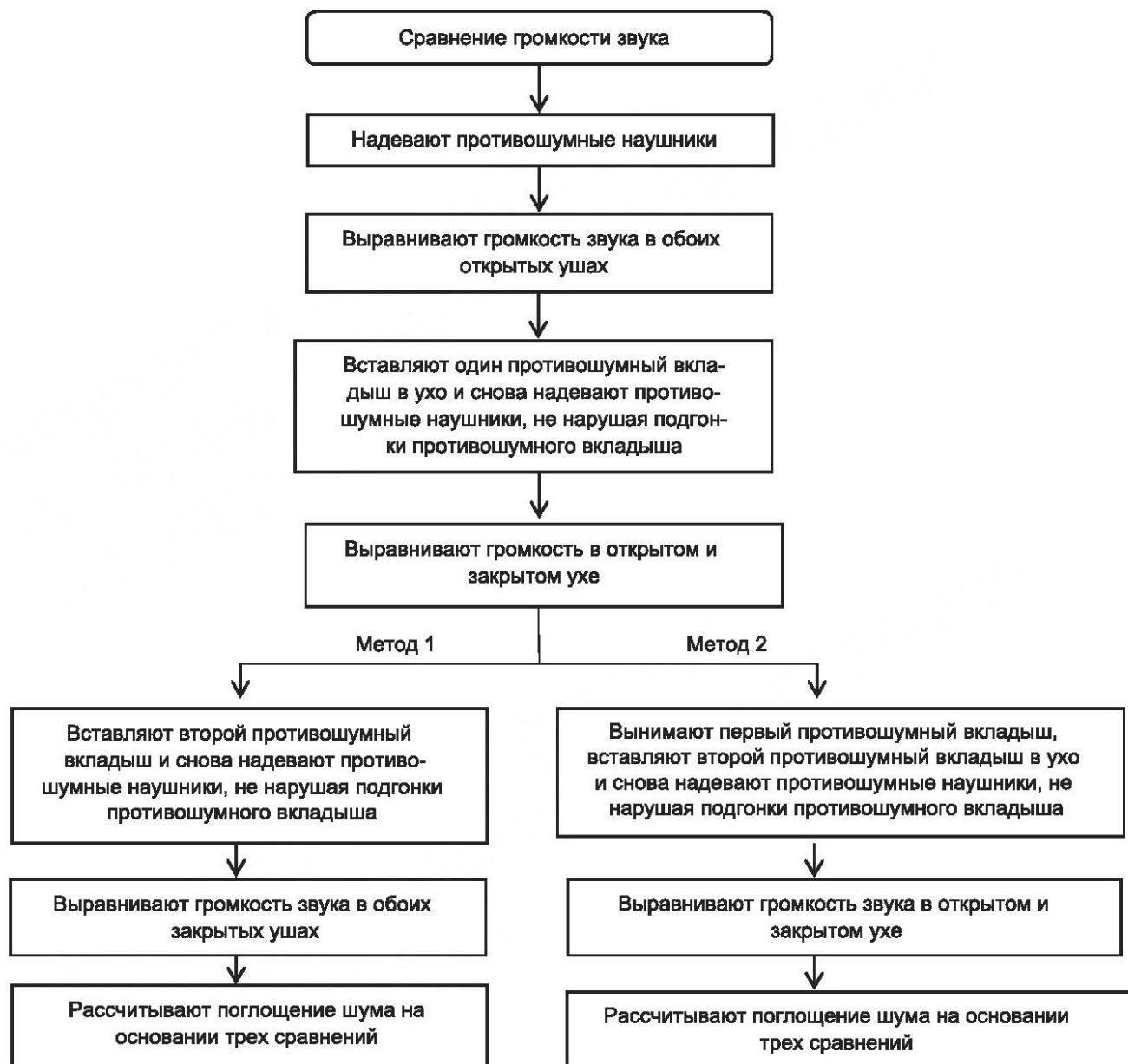
Рисунок 5 — Блок-схема для метода сравнения громкости
