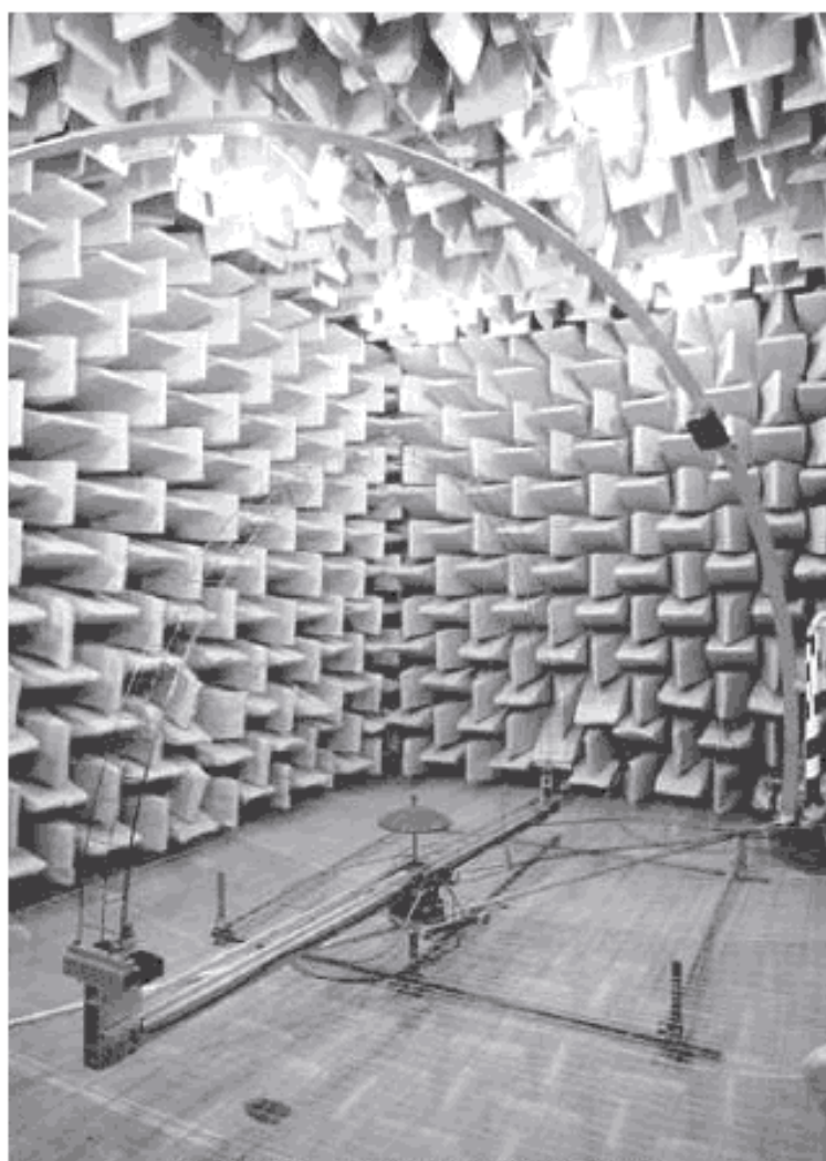
Рисунок 2 – Трехмерный гониометр
