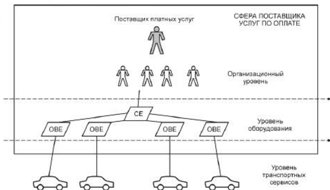
Рисунок 3 — Домен поставщика платных услуг
