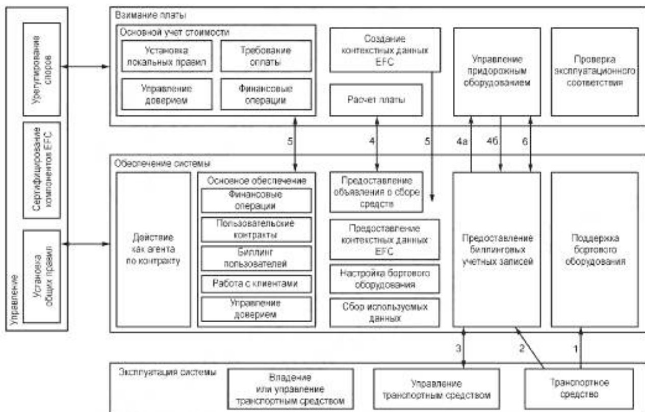
Рисунок D.3 — Подробная ролевая схема EETS
