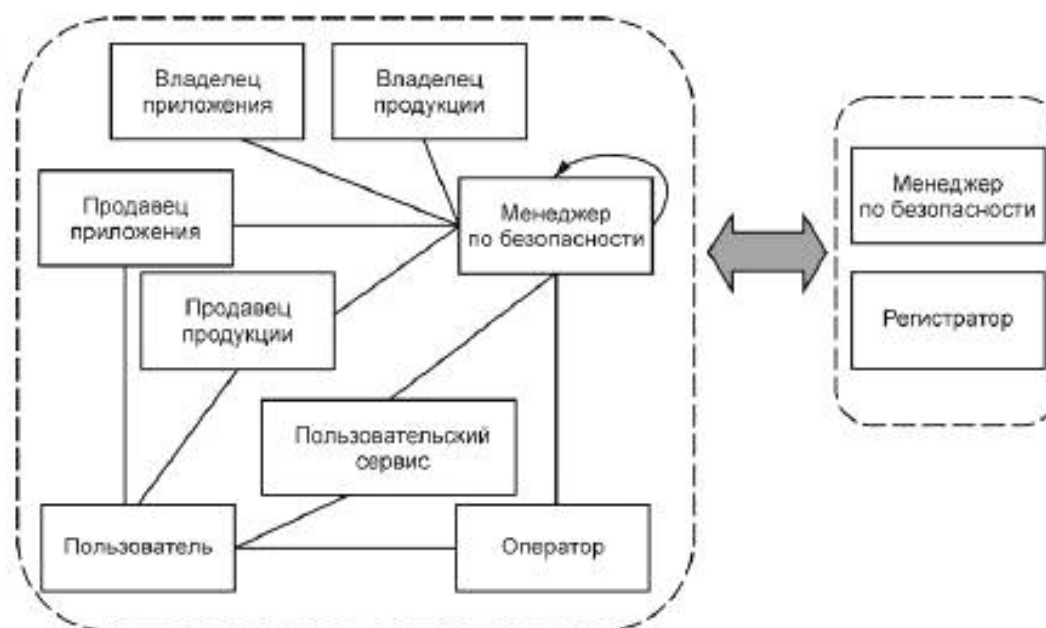
Рисунок С.1 — Концептуальная модель системы
