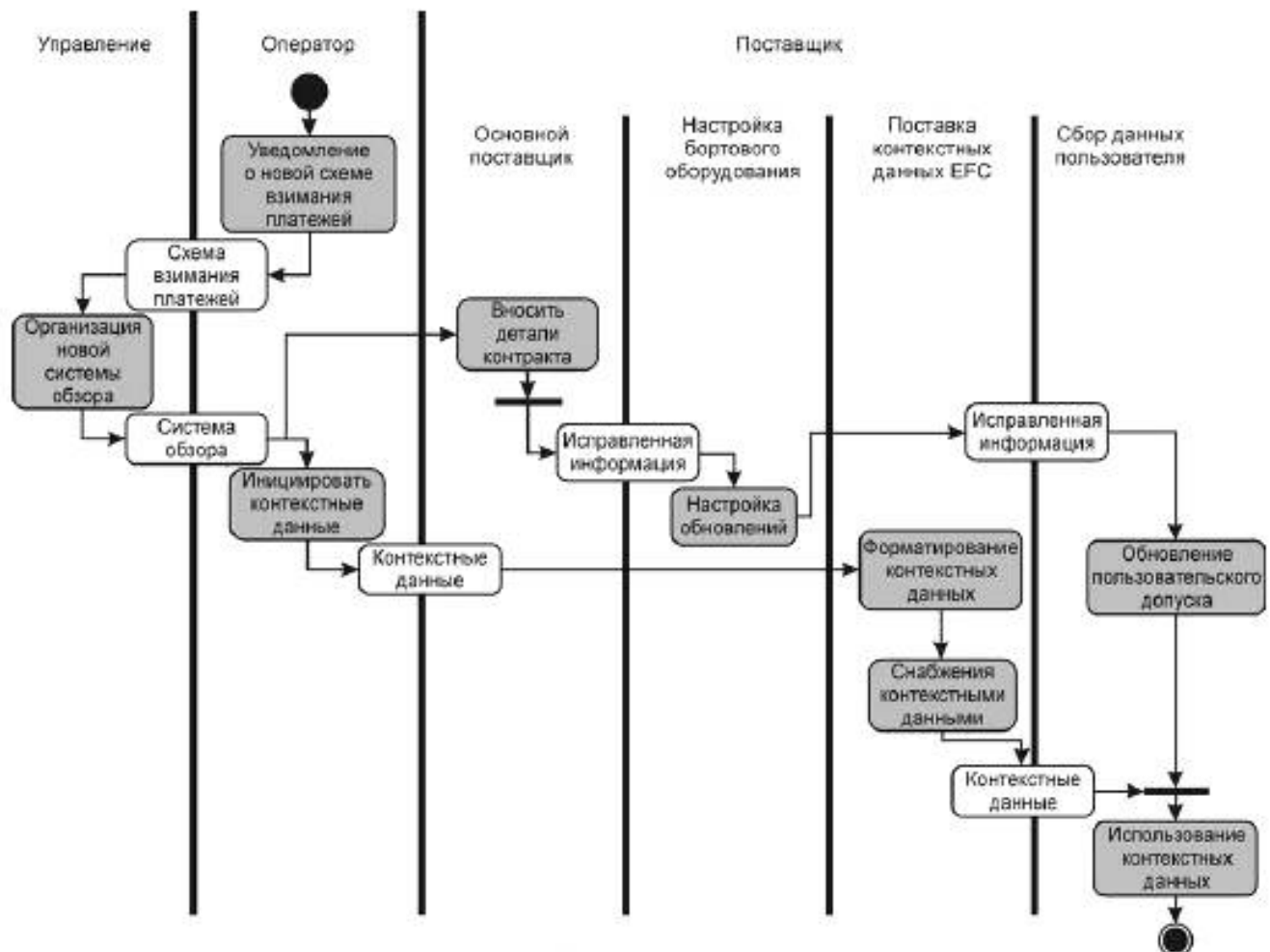
Рисунок 11 — Добавление или модификация режима взимания платы
