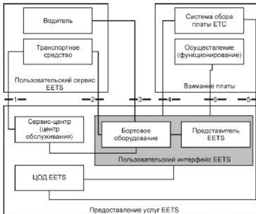
Рисунок D.2 — Архитектура RCI
