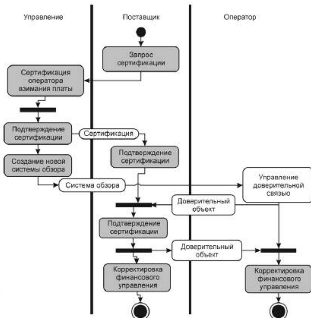
Рисунок 9 — Добавление новых операторов
