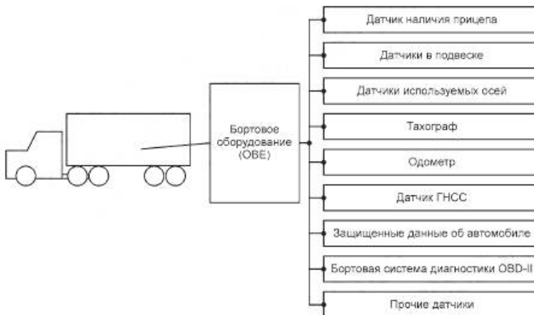
Рисунок 4 — Бортовые устройства и внешние датчики
