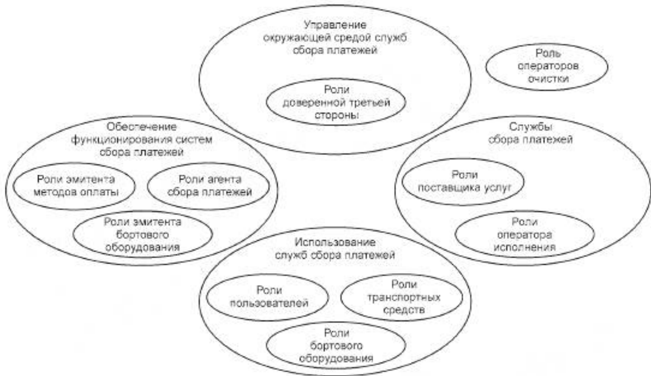
Рисунок E.2 — Роли актеров UML в новой модели
