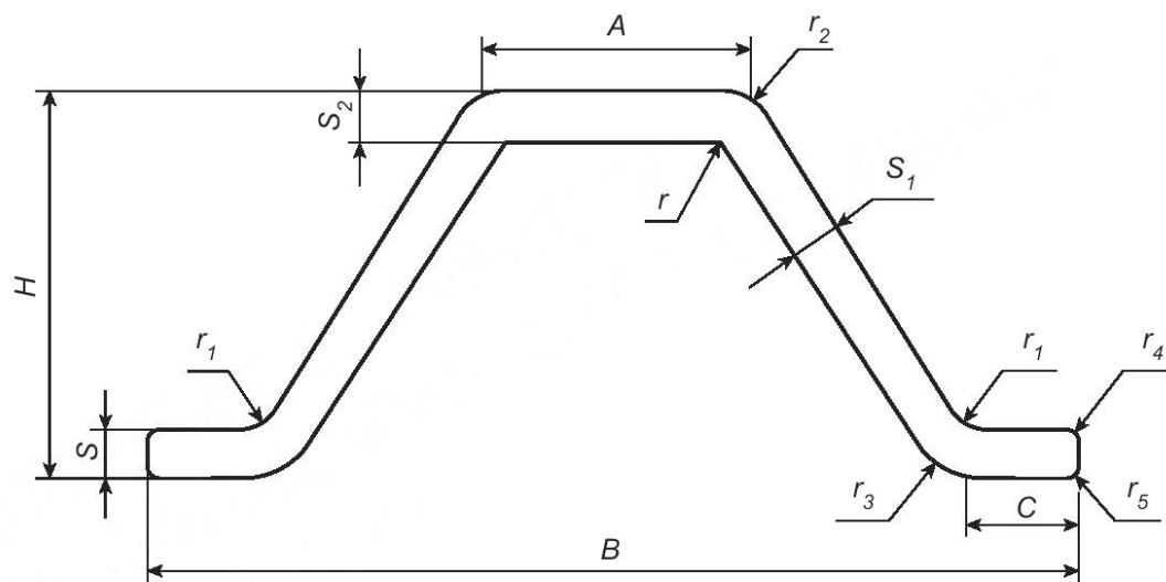
B — длина; A , C — длина полки; H — высота; S , S_1 , S_2 — толщина; r , r_1 , r_2 , r_3 , r_4 , r_5 — радиусы притупления Рисунок 1 — Прессованный косоугольный профиль трапецевидного отбортованного сечения
