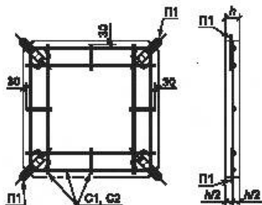
Рисунок Б.2 — Армирование тротуарных плит 7К, 8К
