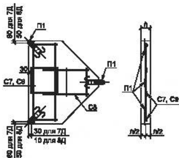
Рисунок Б.5 — Армирование тротуарных плит 7Д, 8Д
