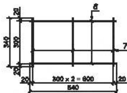
Рисунок Б.12 — Арматурная сетка С10
