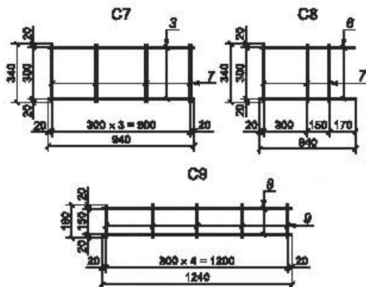
Рисунок Б.11 — Арматурные сетки C7, C8, C9
