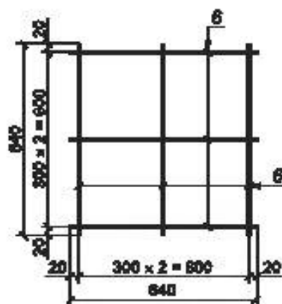
Рисунок Б.10 — Арматурная сетка C6
