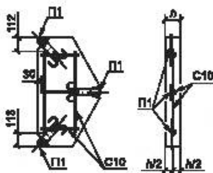
Рисунок Б.6 — Армирование тротуарной плиты 11Д
