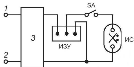
г) Схема включения металлогалогенных и натриевых ламп с импульсным зажигающим устройством (ИЗУ), подключенным последовательно-параллельно
