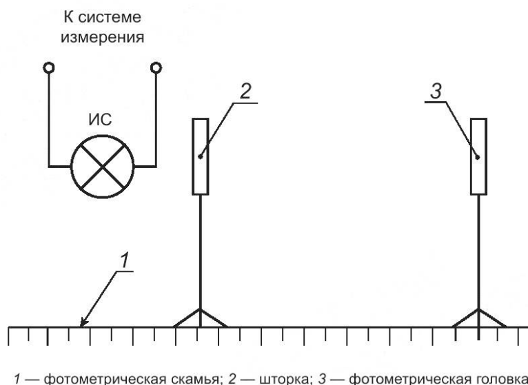
Рисунок В.1 — Схема испытательной установки для проверки утомляемости селеновых фотозадающих элементов
