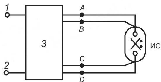
б) Схема включения дуговых ртутных ламп
